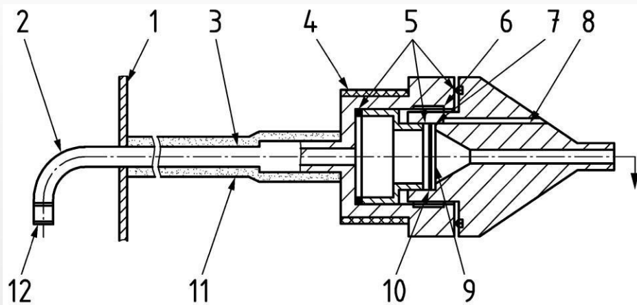
Rysunek A.3 — Propozycja wykonania obudowy filtra PN-EN303-5:2012
