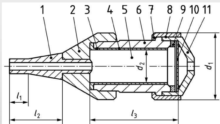
Rysunek A.3 — Propozycja wykonania obudowy filtra PN-EN303-5:2012
