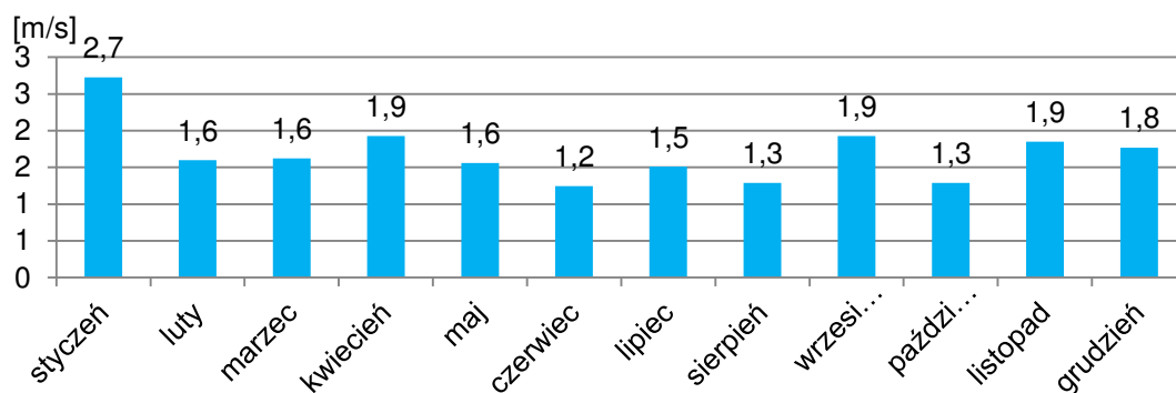
Rysunek 94. Średnie prędkości wiatru w poszczególnych miesiącach 2015 roku w Zakopanem.
