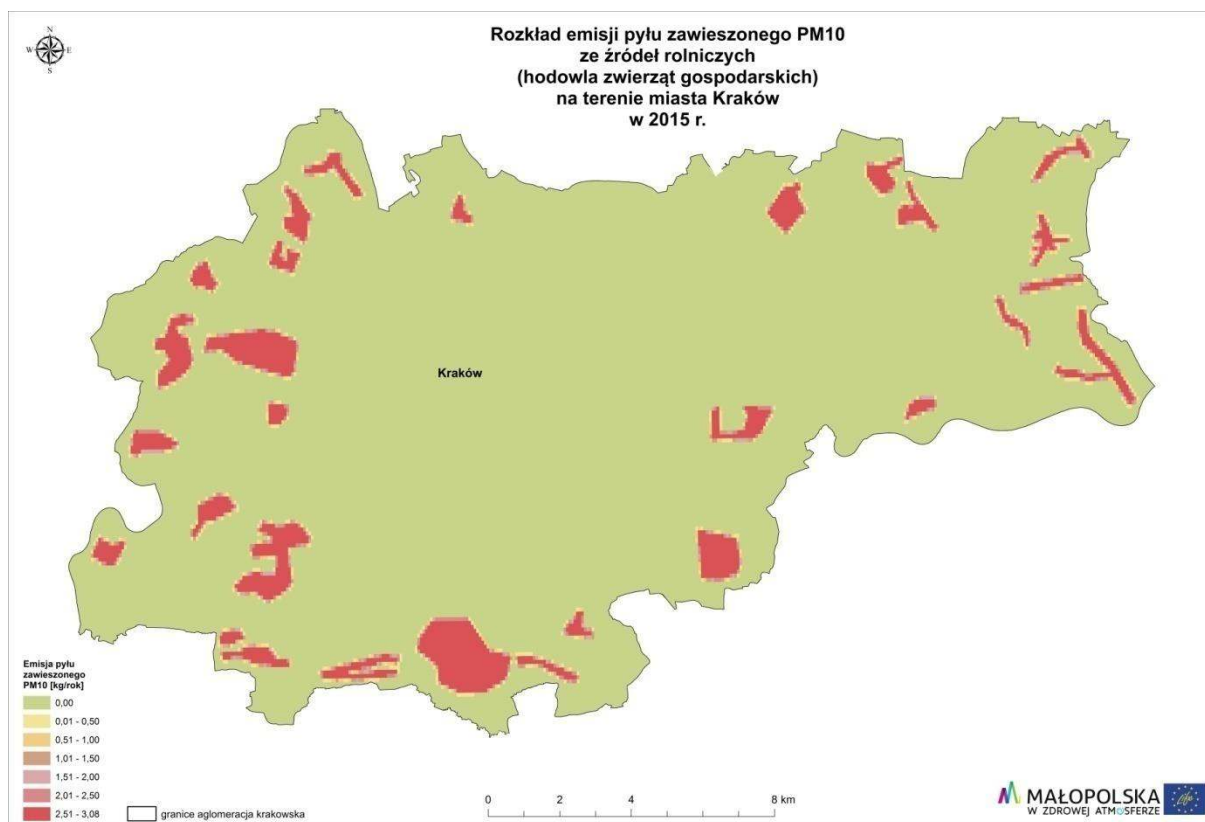
Rysunek 177. Lokalizacja i wielkość emisji pyłu PM10 ze źródeł rolniczych w aglomeracji krakowskiej – hodowla. 172
