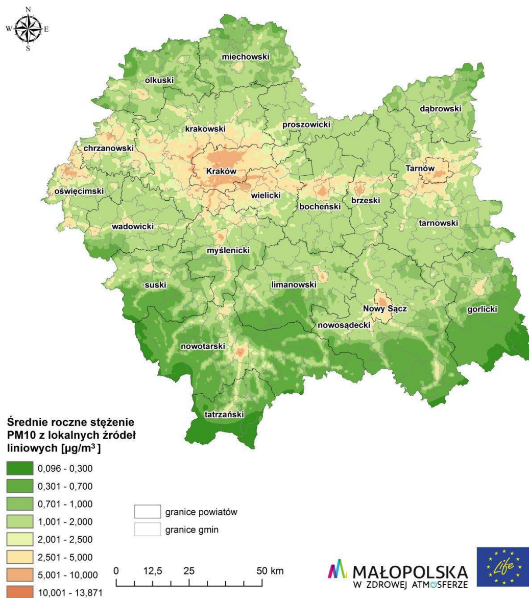
Rysunek 65. Średnie roczne stężenie pyłu PM10 ze źródeł liniowych zlokalizowanych w województwie małopolskim. 53
