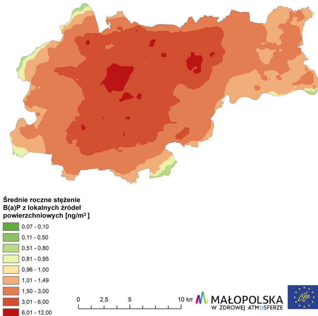
Rysunek 55. Średnie roczne stężenie benzo(a)pirenu ze źródeł powierzchniowych zlokalizowanych w aglomeracji krakowskiej 43
