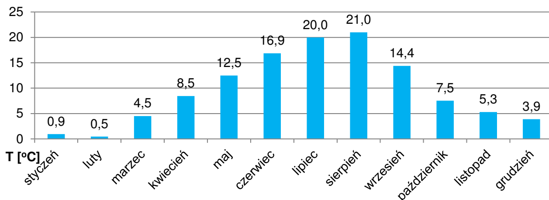
Rysunek 76. Średnie miesięczne temperatury w 2015 roku w Krakowie.
