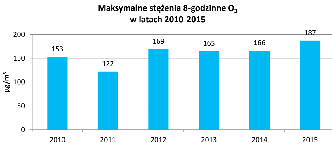
Rysunek 18. Maksymalne 8-godzinne średnie kroczące stężenia ozonu w latach 2010-2015.
