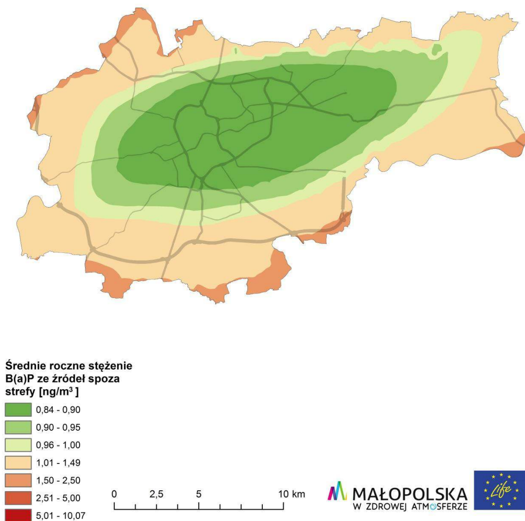
Rysunek 58. Średnie roczne stężenie benzo(a)pirenu ze źródeł zlokalizowanych poza aglomeracją krakowską. 46
