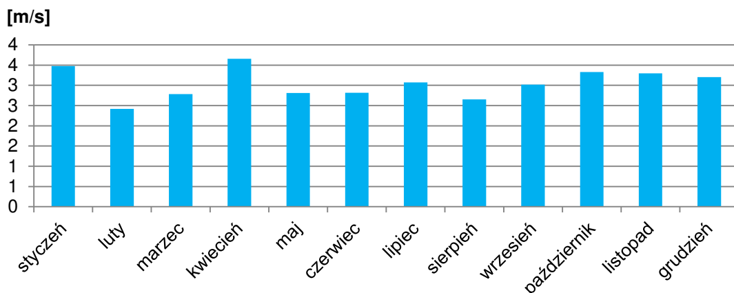
Rysunek 78. Średnie prędkości wiatru w poszczególnych miesiącach 2015 roku w Krakowie.
