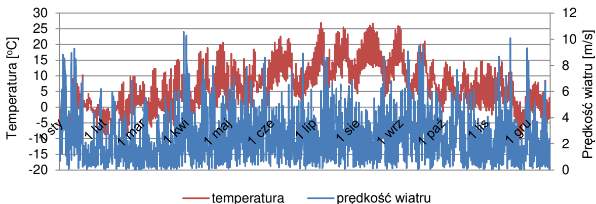
Rysunek 87. Przebieg zmienności temperatury i prędkości wiatru w Nowym Sączu w 2015 roku.
