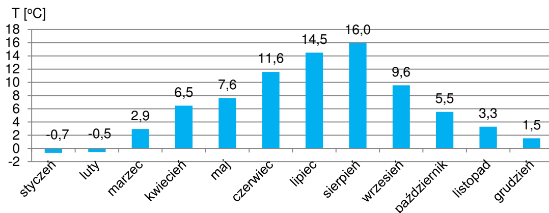
Rysunek 84. Średnie miesięczne temperatury w 2015 roku w Nowym Sączu.
