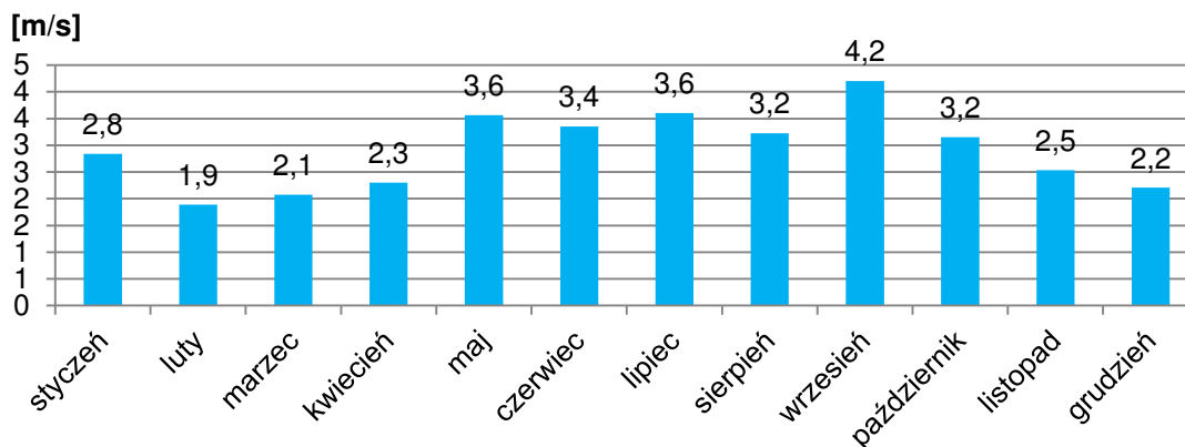
Rysunek 82. Średnie prędkości wiatru w poszczególnych miesiącach 2015 roku w Tarnowie.
