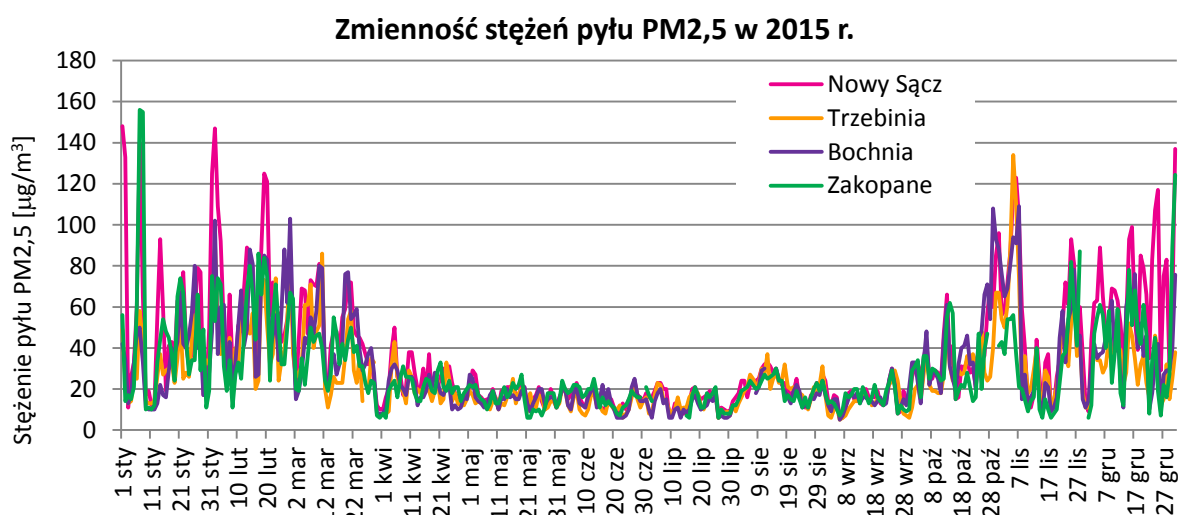
Rysunek 34. Rozkład stężeń pyłu PM 2,5 w roku 2015 na stacjach pomiarowych w strefie małopolskiej.
