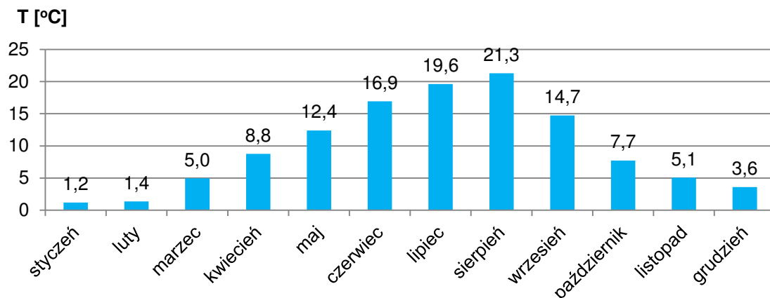
Rysunek 80. Średnie miesięczne temperatury w 2015 roku w Tarnobrzegu.
