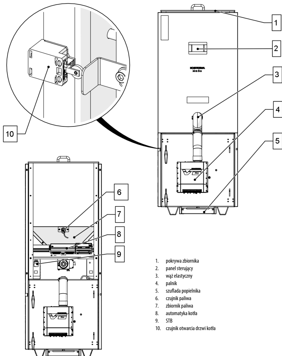
Rysunek : Ogólna budowa kotła EEI Pellets 12kW
