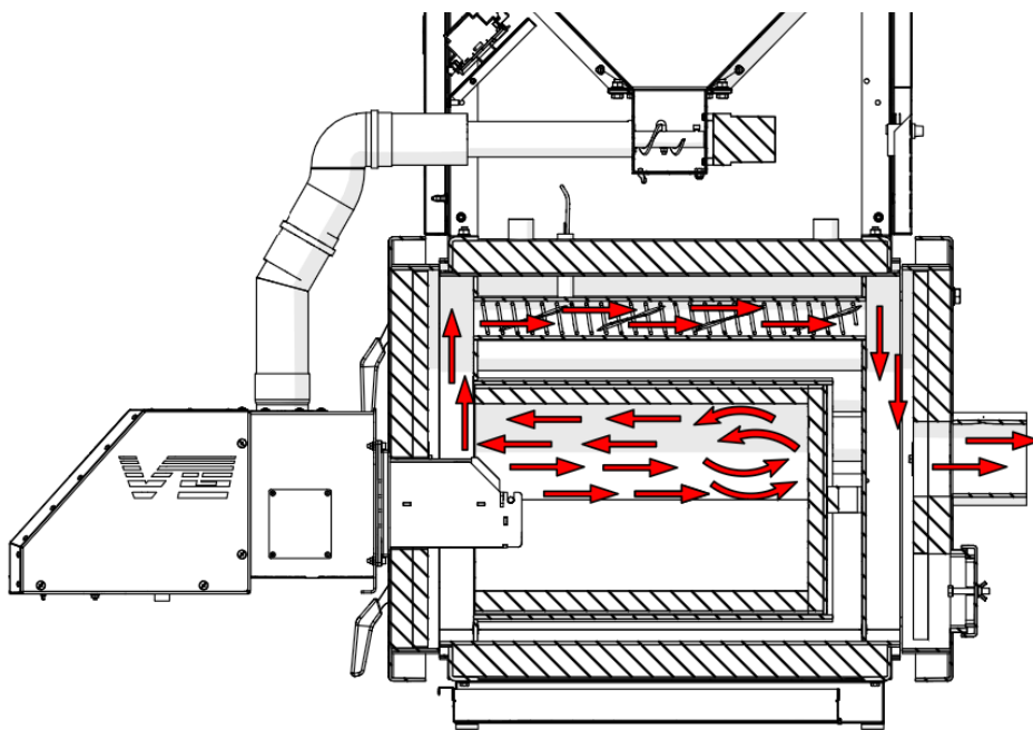
Rysunek : Obieg spalin w kotle EEI Pellets 12kW.
