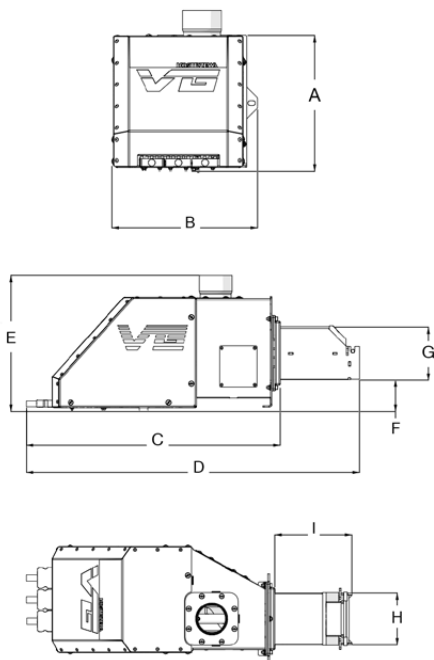
Rys: Schemat wymiarowy palnika Platinum Bio VG 12kW.
