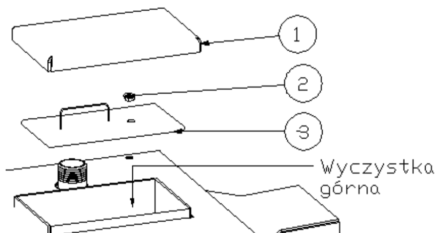
Rys. 8 Czyszczenie kotła przez wyczystkę górną
