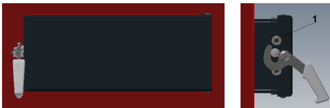
Rys. 16 Mocowanie drzwiczek do ramki kotła (prawie)
