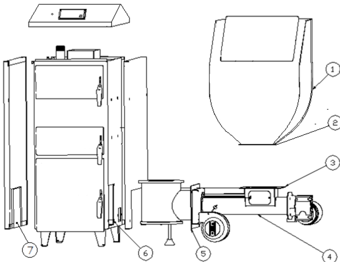
Rys. 11 Przekładanie podajnika na drugą stronę kotła
