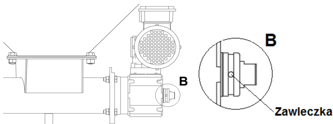
Rys. 7 Sposób montażu zawlecзки motoreduktora ze ślimakiem
