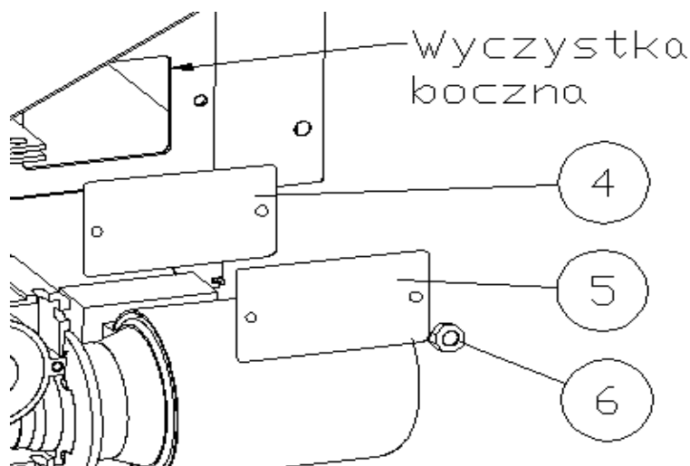
Rys. 9 Czyszczenie kotła przez wyczystkę boczną
