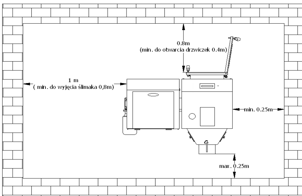
Rys. 2 Usytuowanie kotła w kotłowni
