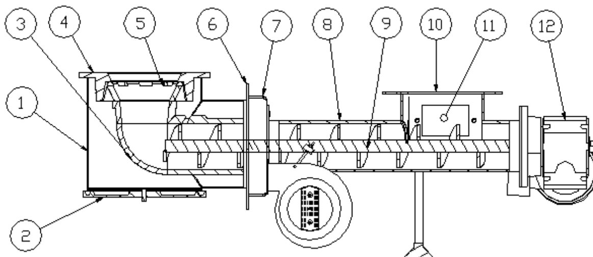
Rys 6 Budowa podajnika paliwa stałego
