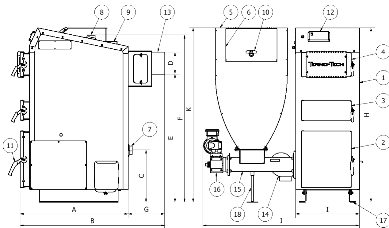
Rys. 1 Wymiary i opis kotła.
