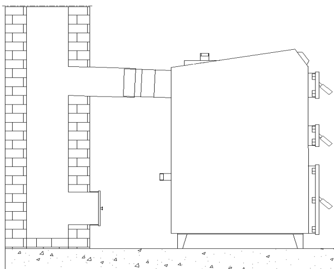
Rys. 3 Podłączenie kotła do komina
