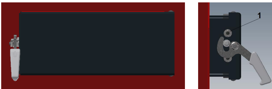
Rys. 16 Mocowanie drzwiczek do ramki kotła (prawe)
