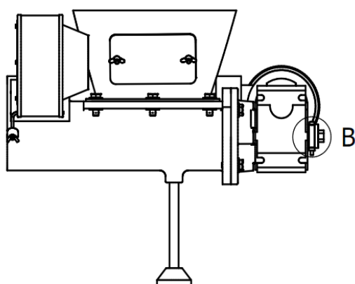
Rys. 7 Sposób montażu zawleczonego motoreduktora ze ślimakiem
