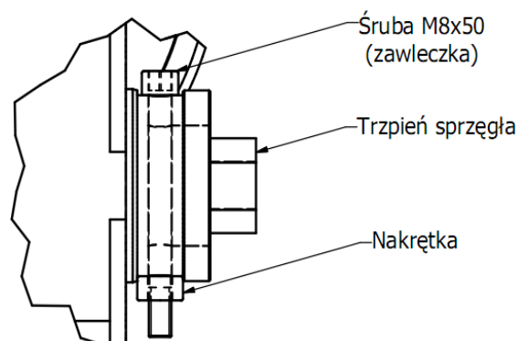
Rys. 7 Sposób montażu zawleczonego motoreduktora ze ślimakiem
