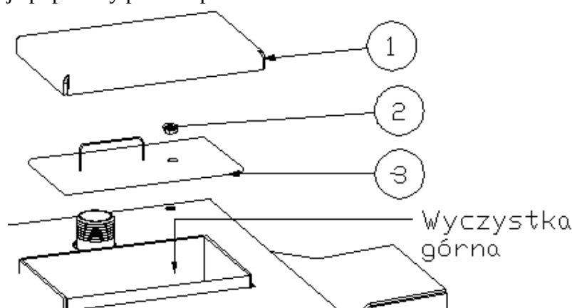
Rys. 9 Czyszczenie kotła przez wyczystkę górną
