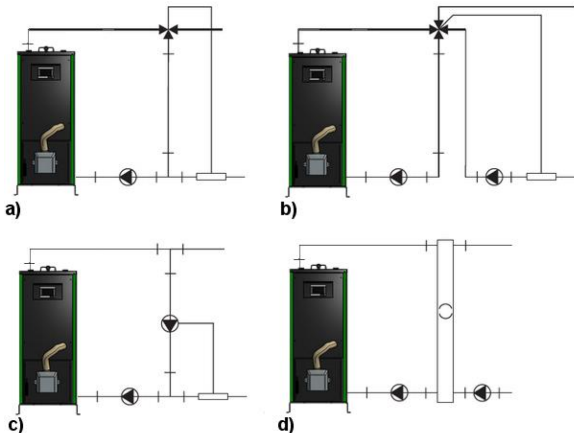
Rys. 4. Zalecane możliwe schematy połączenia kotła KAMEN z instalacją grzewczą: a) z zaworem trójdrożnym; b) z zaworem czterodrożnym; c) z pompą przevalową; d) ze sprzęgłem hydraulicznym
