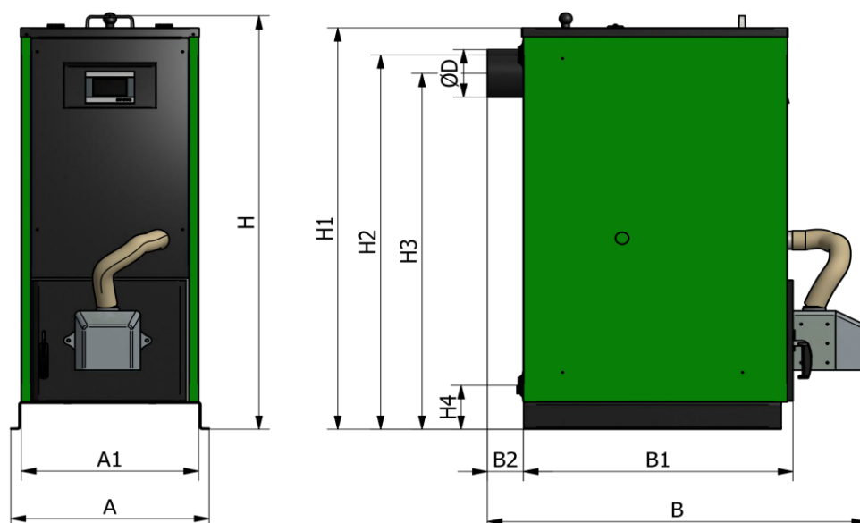
Rys 2. Podstawowe wymiary kotła Kamen PERFEKT Bio.
