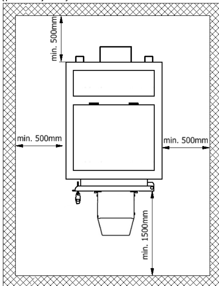
Rys 3. Ustawienie kotła KAMEN w pomieszczeniu kotłowni.
