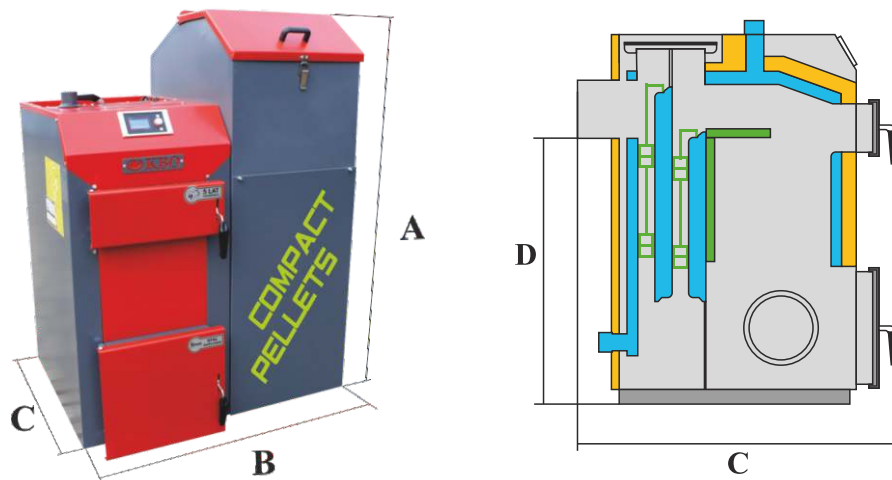
Rys. 1 Przekrój kotła
