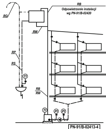
Rysunek 4. Schemat zabezpieczenia instalacji ogrzewania wodnego, wyposażonej w jeden kocioł lub wymiennik ciepła, rozdzielacz, pompa zamontowana na powrocie. Schemat zabezpieczenia ma również zastosowanie do następujących instalacji ogrzewania wodnego:
