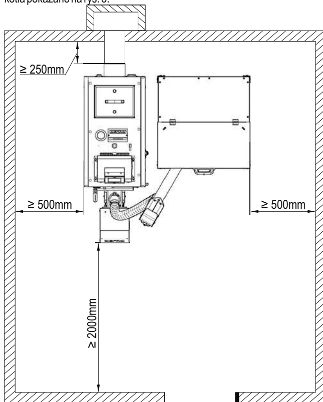
Rysunek 3. Ustawienie kotła w pomieszczeniu kotłowni.
