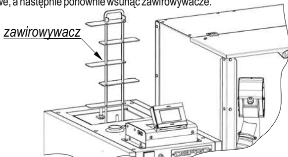
Rysunek 19. Zawirówkę w kotle.
