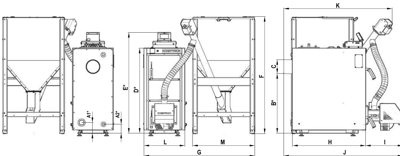
Rysunek 1. Podstawowe wymiary kotłów.
