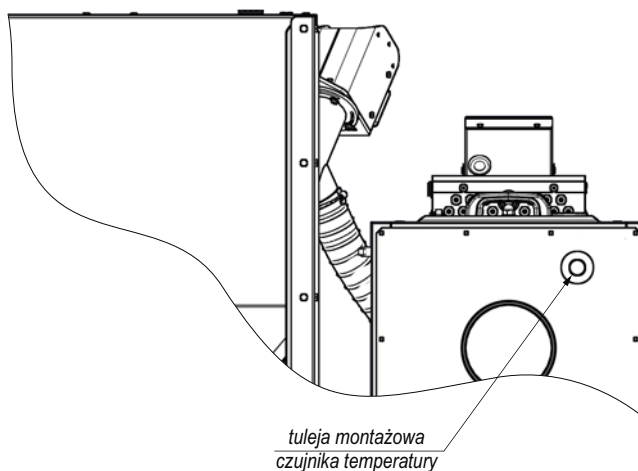
Rysunek 8. Sposób podłączenia czujnika temperatury.
