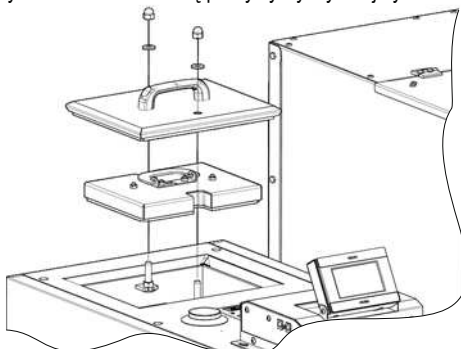
Rysunek 20. Sposób demontażu pokryw wyczystnej.
