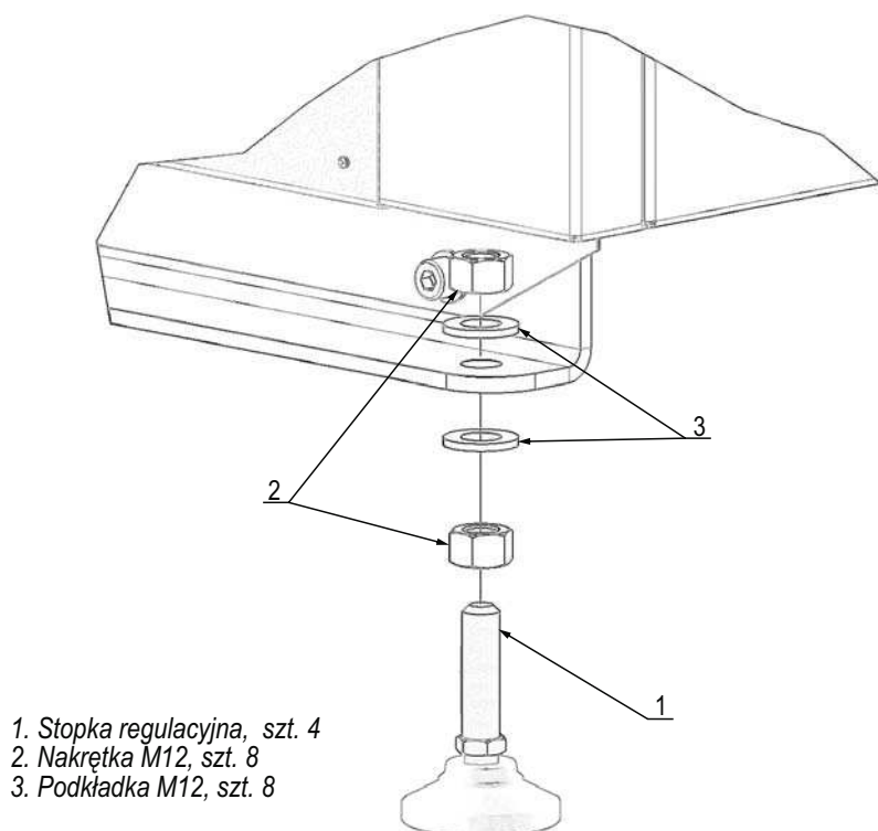
Rysunek 21. Sposób montażu stopek ustalających kocioł.
