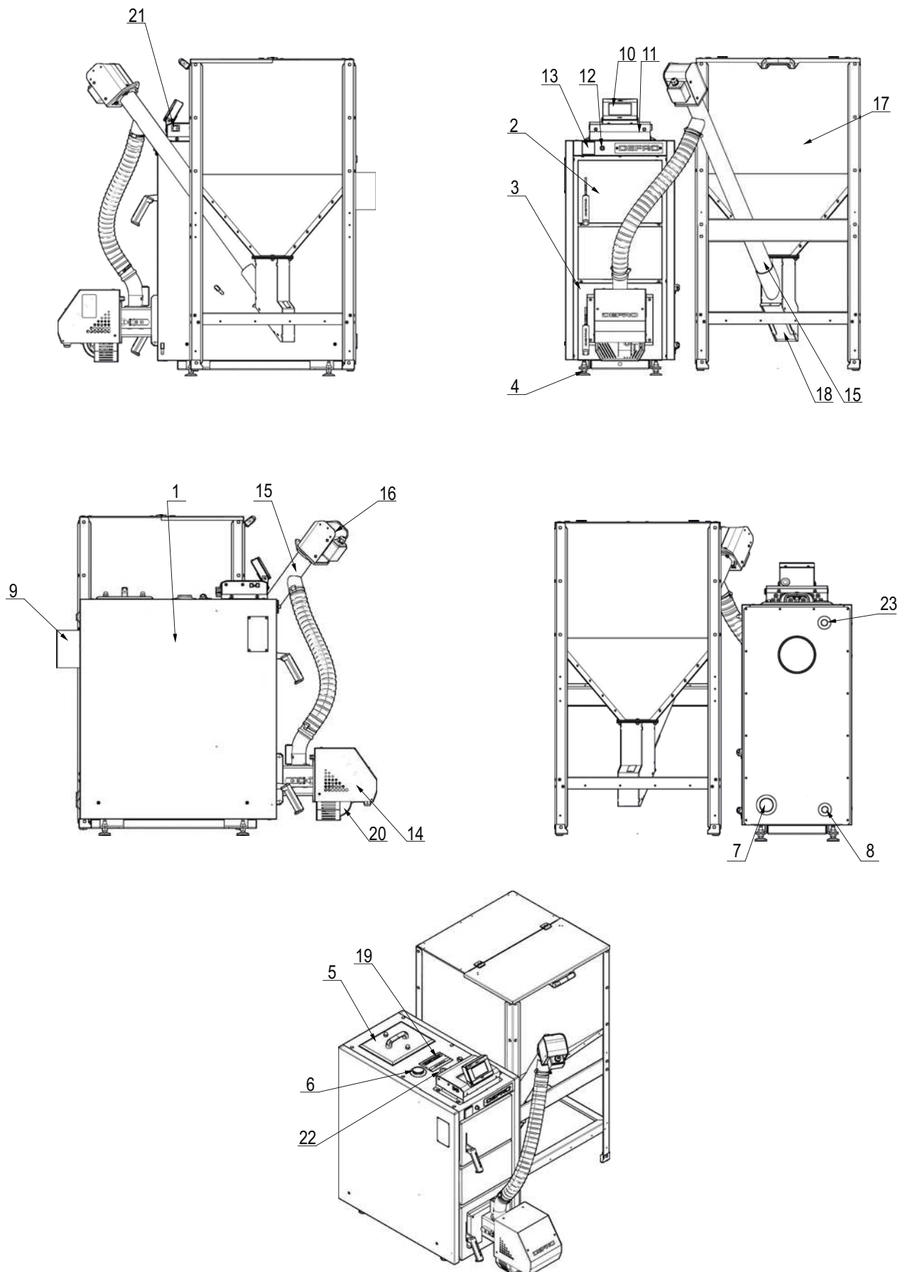
Rysunek 2. Podstawowe elementy kotłów: 1-korpus stalowy z izolacją termiczną; 2-drzwi wyczystne; 3-drzwi paleniskowo-popielnikowe; 4-stopki do poziomowania kotłów; 5-wyczystka górna; 6-króciec zasilający; 7-króciec powrotny; 8-króciec spustowy; 9-czopuch; 10-wyświetlacz regulatora elektronicznego; 11- moduł sterujący; 12-ogranicznik temperatury STB; 13-termometr analogowy; 14-palnik pelletowy; 15-podajnik paliwa; 16-motoreduktor; 17-zasobnik paliwa; 18-otwór rewizyjny zasobnika paliwa; 19-maskownica tulei montażowych czujników sterownika; 20-wentylator; 21-wyłącznik główny; 22-przelotka przewodu czujnika spalin; 23-króciec 1/2" (do montażu czujnika temperatury zabezpieczenia SYR 5067).
