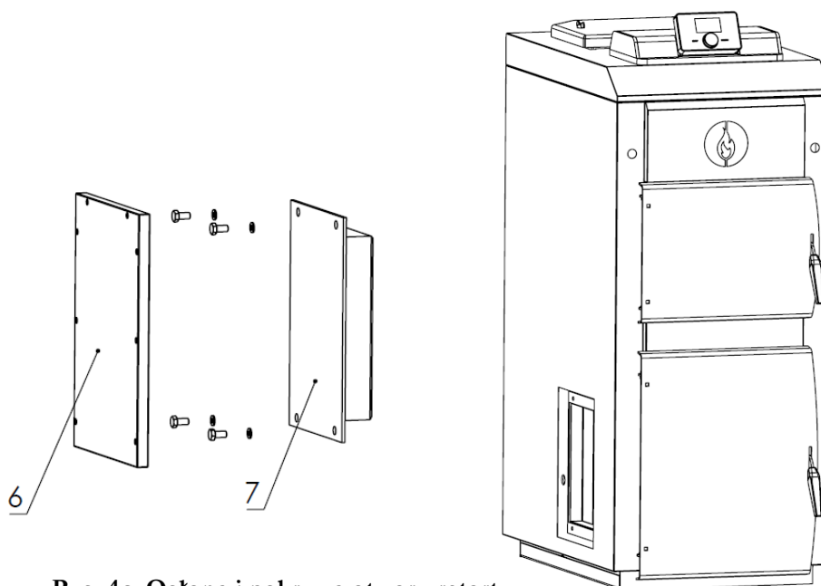
Rys. 4c. Osłona i pokrywa otworu retorty.
