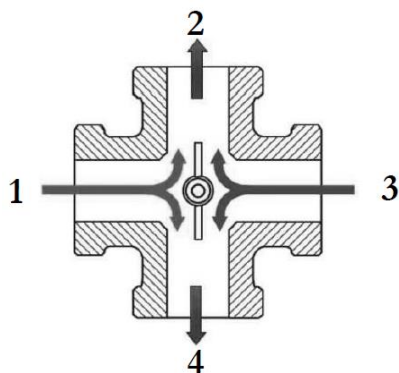
Rys. 10. Czterodrożny zawór mieszający
