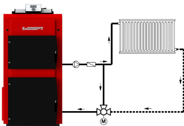
Rys. 11a. Przykład montażu zaworu mieszającego w instalacji z regulacją ilościową (zapewnia ochronę kotła przed „zimnym” powrotem czynnika grzewczego).
