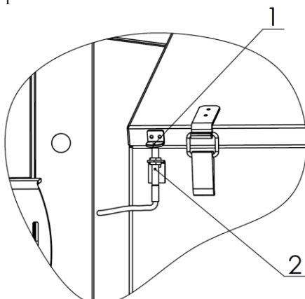
Rys. 6. Wyłącznik bezpieczeństwa klapy zasobnika.
