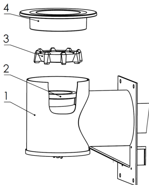
Rys. 14a. Demontaż palnika retortowego
