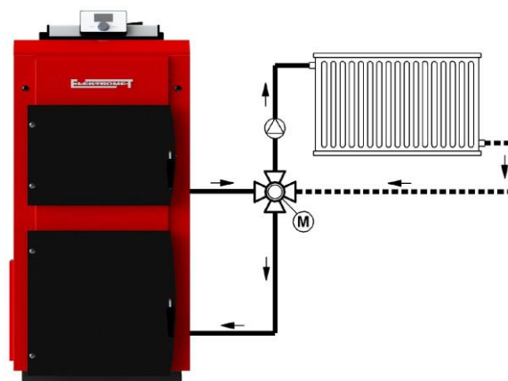
Rys.10a. Przykład montażu zaworu mieszającego czterodrożowego.
