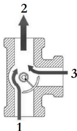
◀ Rys. 11. Trójdrożny zawór mieszający
