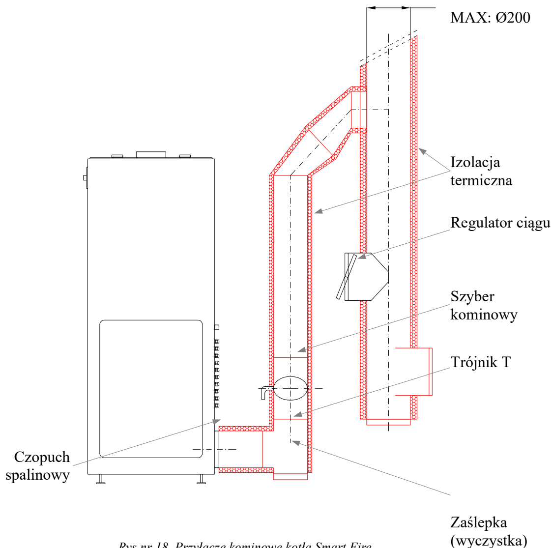
Rys nr 18. Przyłącze kominowe kotła Smart Fire
