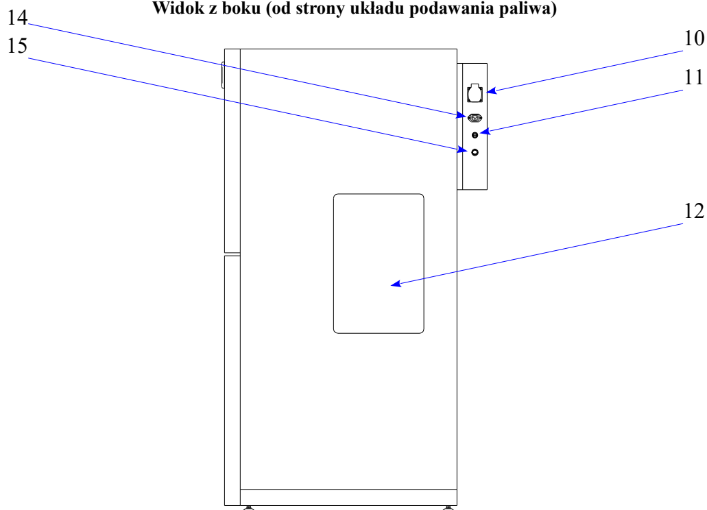
Rys nr 10. Opis schematyczny kotła Smart Fire SF11/130L
