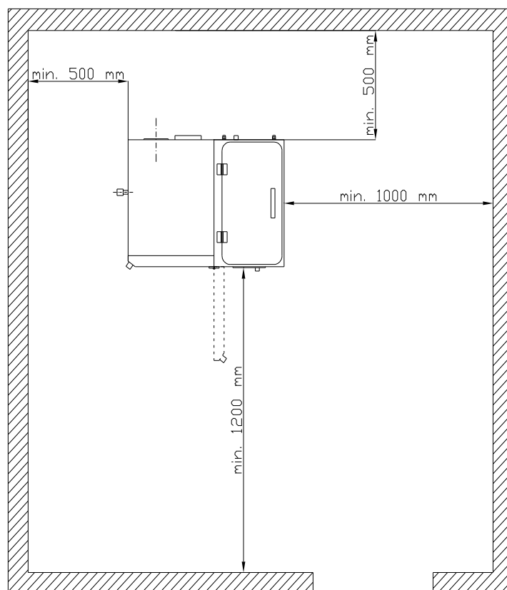
Rys nr 17. Przykład umiejscowienia kotła Smart Fire w kotłowni
