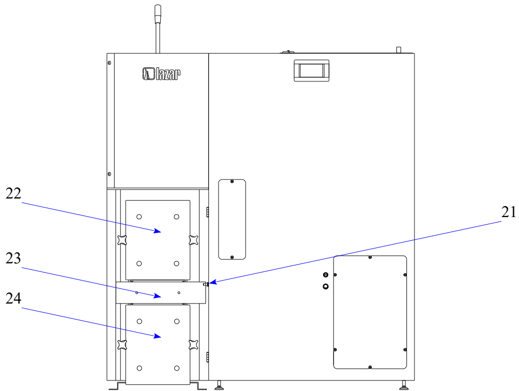
Rys nr 7. Opis schematyczny kotłów typu Smart Fire SF 11, SF15, SF22, SF31 oraz SF41
