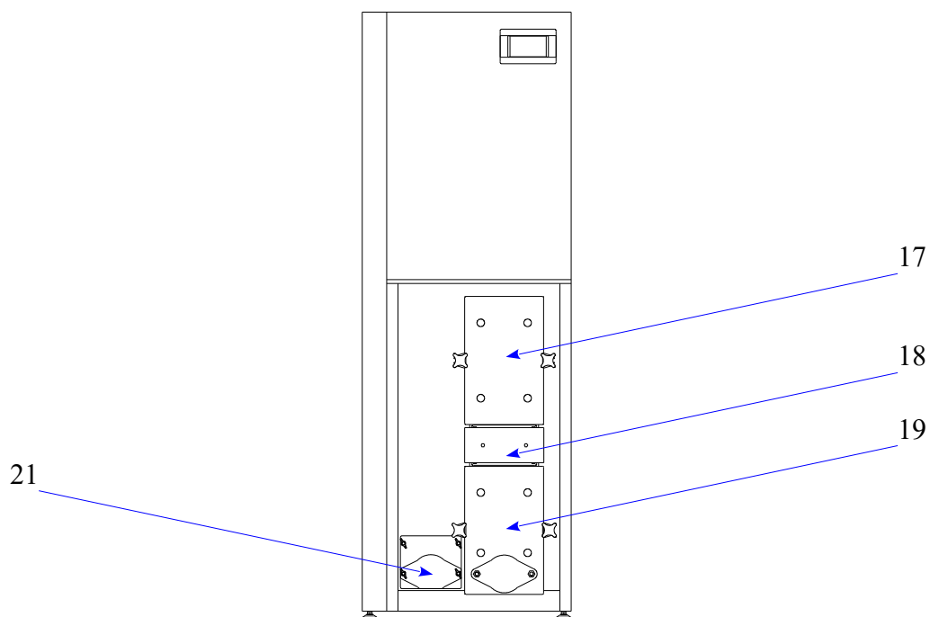
Rys nr 11. Opis schematyczny kotła Smart Fire SF11/130L
