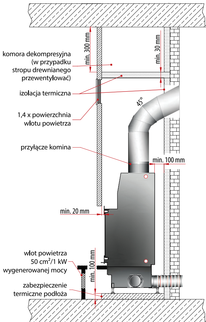
Rys. 3. Schemat przyłączenia wkładu Unico do kominika.
