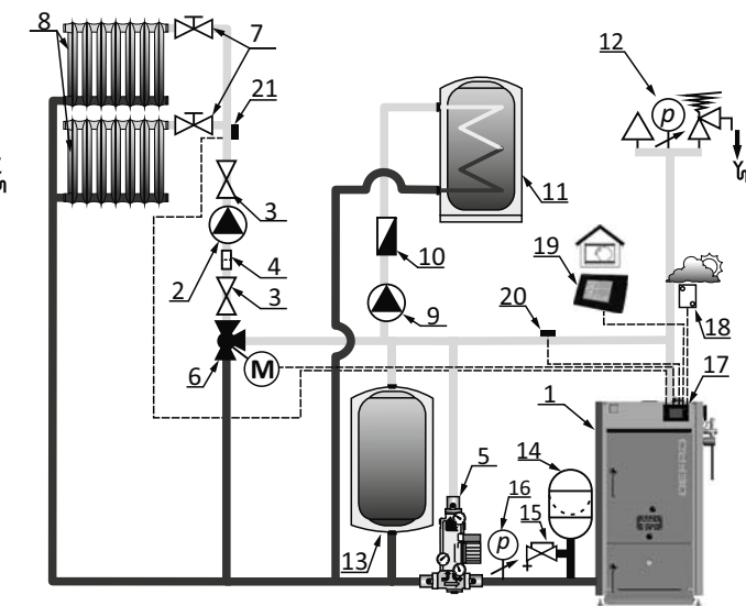
1-kocioł; 2-pompa c.o.; 3-zawór odcinający; 4-filtr; 5-ladomat; 6-zawór 3-drogowy mieszający; 7-zawór z głowicą termostatyczną; 8-grzejnik; 9-pompa c.w.u.; 10-zawór zwrotny; 11-zasobnik c.w.u.; 12-grupa bezpieczeństwa; 13-zbiornik akumulacyjny; 14-naczynie przeponowe; 15-zawór kółpakowy; 16-manometr; 17-termoregulator /sterownik zaworu mieszającego/; 18-sterownik pokojowy 19-czujnik temperatury pogodowy; 20-czujnik temperatury zasilania; 21-czujnik temperatury CO
