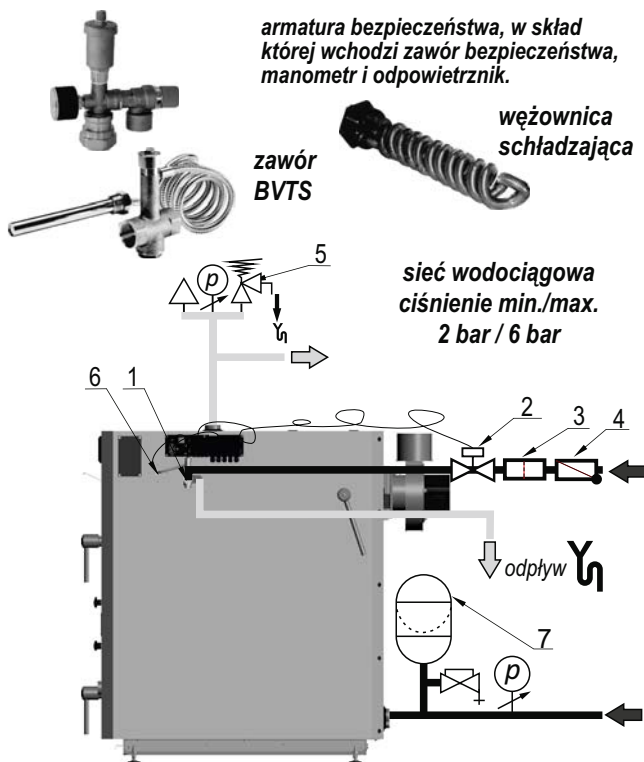
Rysunek 8. Przykładowy schemat zabezpieczeń instalacji ogrzewania wodnego w kotle DEFRO HG
