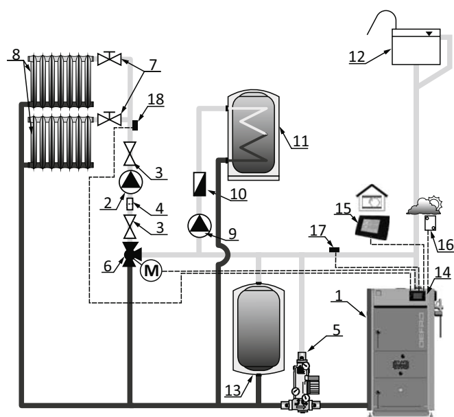
1-kocioł; 2-pompa c.o.; 3-zawór odcinający; 4-filtr; 5-ladomat; 6-zawór 3-drogowy mieszający; 7-zawór z głowicą termostatyczną; 8-grzejnik; 9-pompa c.w.u.; 10-zawór zwrotny; 11-zasobnik c.w.u.; 12-otwarte naczynie wzbiorcze; 13-zbiornik akumulacyjny; 14-termoregulator /sterownik zaworu mieszającego/; 15-sterownik pokojowy 16-czujnik temperatury pogodowy; 17-czujnik temperatury zasilania; 18-czujnik C.O.
