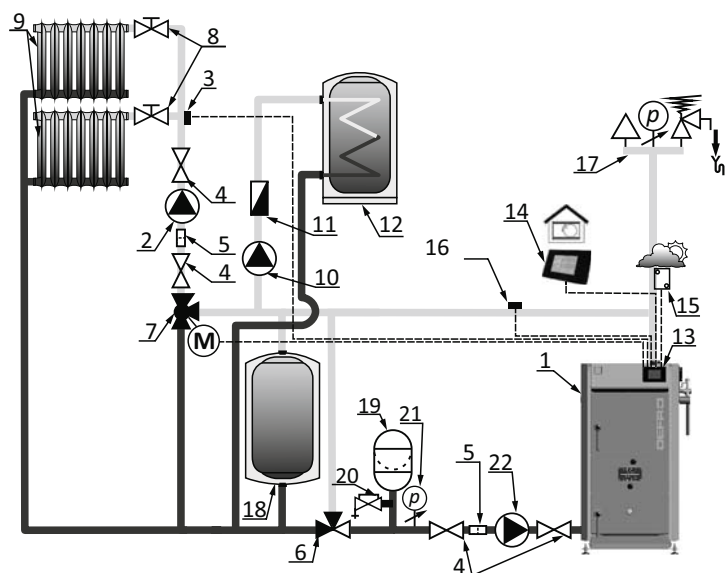
1-kocioł; 2-pompa c.o.; 3-czujnik c.o.; 4-zawór odcinający 5-filtr; 6-zawór termostatyczny min 55°C; 7-zawór 3-drogowy mieszający 8-zawór z głowicą termostatyczną; 9-grzejnik; 10-pompa c.w.u. 11-zawór zwrotny; 12-zasobnik c.w.u.; 13-termoregulator /sterownik zaworu mieszającego/; 14-sterownik pokojowy 15-czujnik temperatury pogodowy; 16-czujnik temperatury zasilania; 17-grupa bezpieczeństwa; 18-zbiornik akumulacyjny 19-naczynie przeponowe; 20-zawór kółpakowy; 21-manometr; 22-pompa by-pass.
