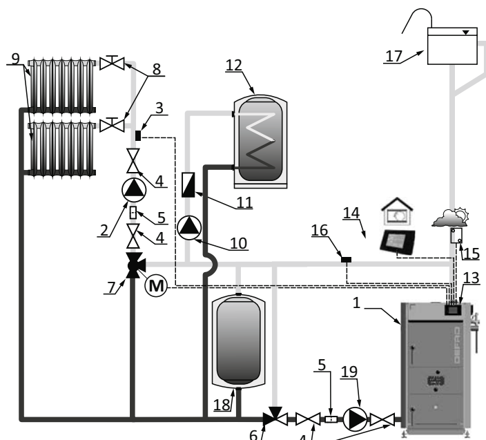
1-kocioł; 2-pompa c.o.; 3-czujnik c.o.; 4-zawór odcinający 5-filtr; 6-zawór termostatyczny min 55°C; 7-zawór 3-drogowy mieszający 8-zawór z głowicą termostatyczną; 9-grzejnik; 10-pompa c.w.u. 11-zawór zwrotny; 12-zasobnik c.w.u.; 13-termoregulator /sterownik zaworu mieszającego/; 14-sterownik pokojowy 15-czujnik temperatury pogodowy; 16-czujnik temperatury zasilania; 17-otwarte naczynie wzbiorcze; 18-zbiornik akumulacyjny; 19 - pompa by-pass.
