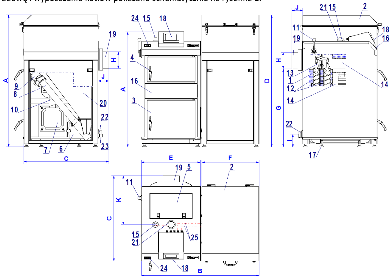
WYMIARY KOTŁOW Setlans BIOFUEL [mm]
