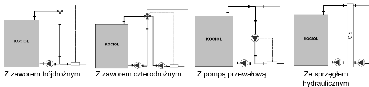
Rys. 5. Zalecane schematy połączeń kotła do instalacji grzewczej
