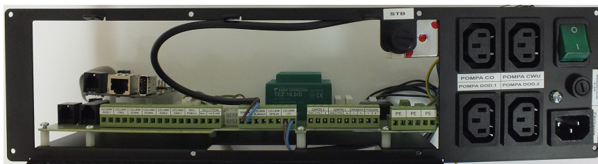
Rysunek 2 Listwa przyłączeniowa do zasilania urządzeń regulacyjnych (uwaga fot. przedstawia przykładowe rozmieszczenie połączeń, szczególnie w dołączonej DTR sterownika).
