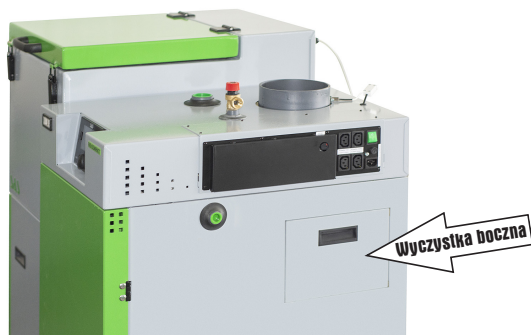
Rysunek 14 Wyczystka boczna w kotle SAS BIO COMPACT (CG) - wersja z czopuchem do góry
