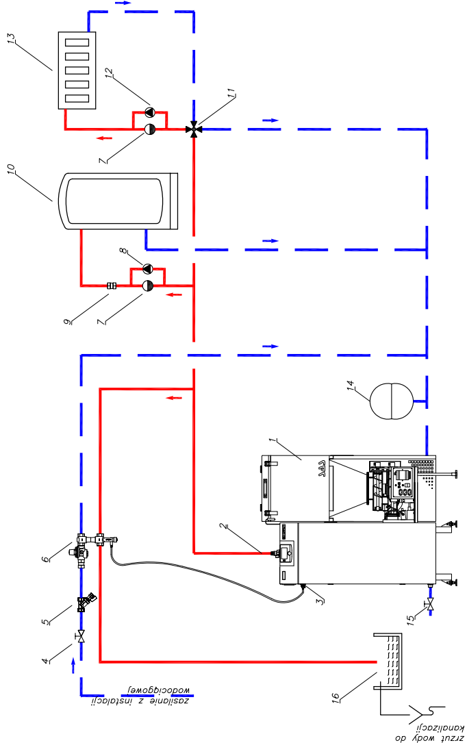
Rysunek. 13. Schemat ogólny podłączenia kotła typu SAS BIO COMPACT do instalacji c.o. i c.w.u. Kocioł w układzie zamkniętym, zabezpieczony przed przegrzaniem zaworem termostatycznym SYR typ 5067
