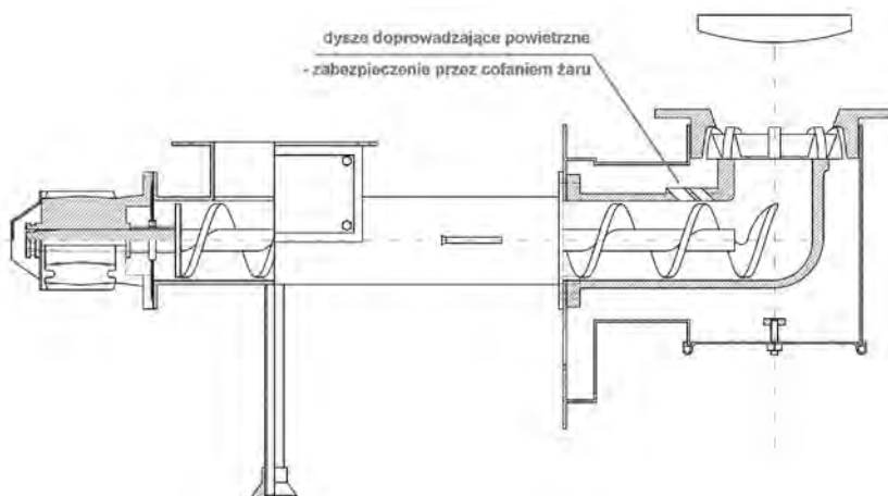
Rysunek 12 Retorta z dyszami powietrznymi w kolanie zabezpieczającymi przez cofaniem żaru.
