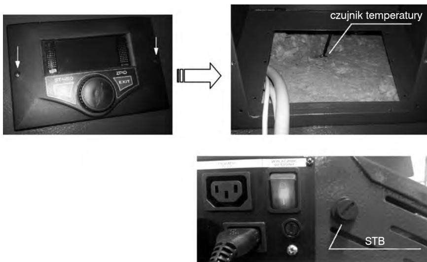
Rysunek 11 Lokalizacja ogranicznika temperatury bezpieczeństwa STB oraz czujnika temperatury
