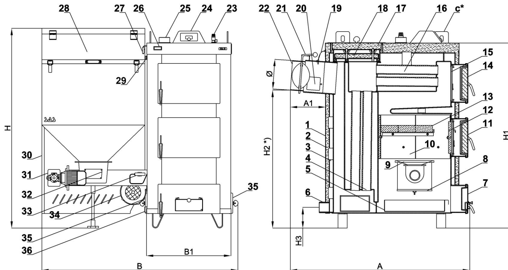
RYSUNEK.4 SCHEMAT KONSTRUKCJI KOTŁA SAS SOLID O MOCY CIEPLNEJ 72 ÷ 200 kW
