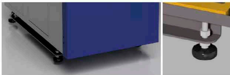
Rys. 2. Stopka regulacyjna, służąca do wypoziomowania kotła typu DWOREK COMFORT BLUE
