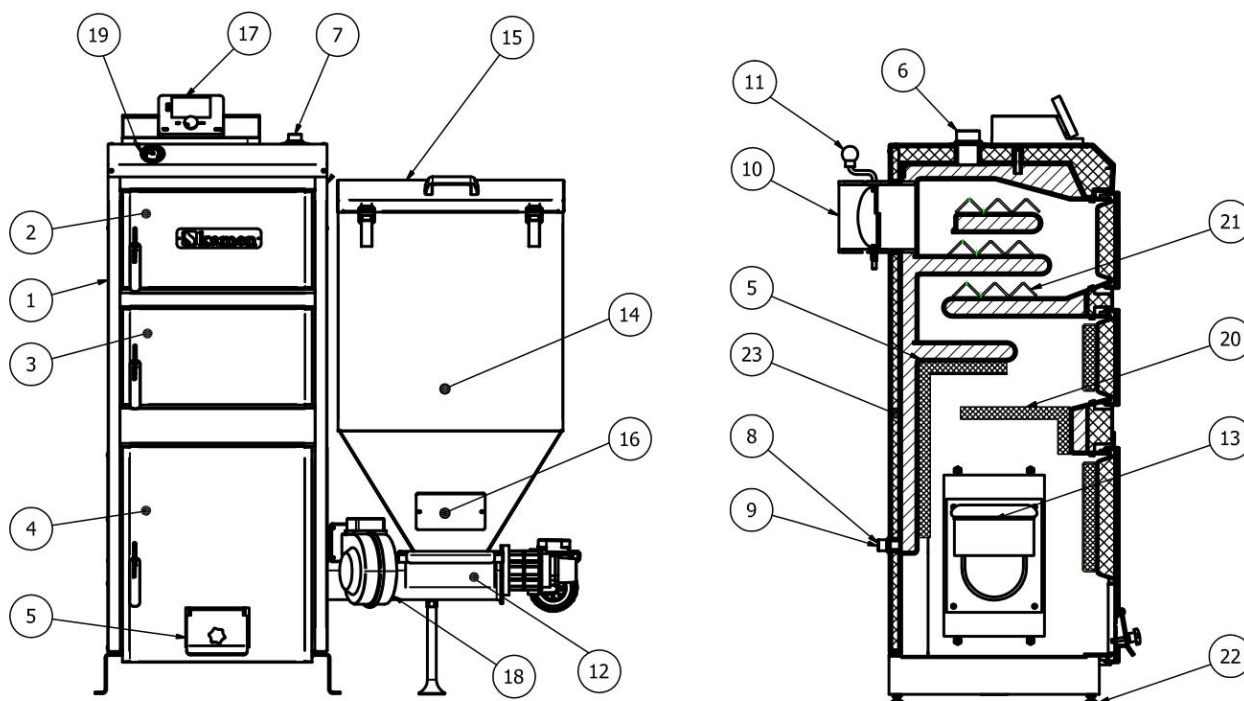
Rys 1. Schemat kotła Kamen MULTI K5 (podstawowe elementy kotła + przekrój).
