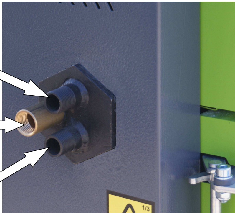
Rys. 2.6.3. Zamontowana wężownica schładzająca, instrukcja podłączenia zaworu termostatycznego JBV1.
