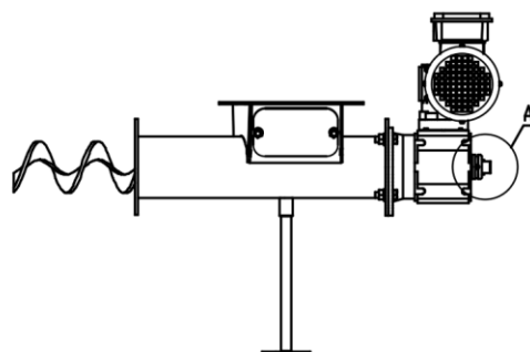
Rys. 7 Sposób montażu zawleczone motoreduktora ze ślimakiem
