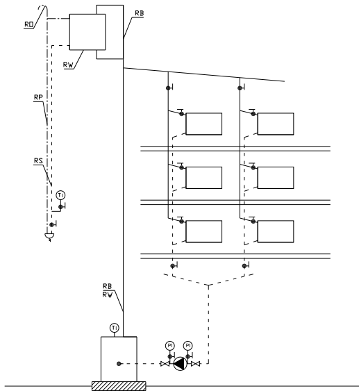
PN-91/B-02413 Schemat zabezpieczenia instalacji ogrzewania wodnego, wyposażonej w jeden kocioł lub wymiennik ciepła, rozdziel górny, pompa zamontowana na powrocie.
