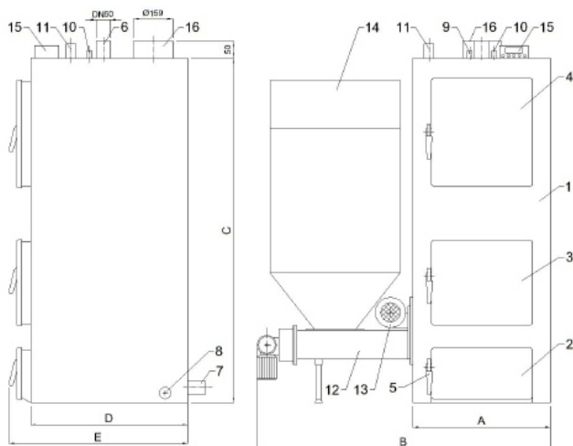
Rys.1. Kocioł „EKO 5S”
