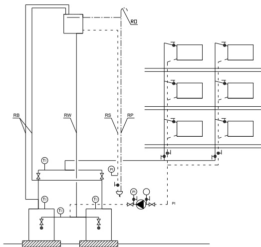
PN-91/B-02413 Schemat zabezpieczenia instalacji ogrzewania wodnego, wyposażonej w dwa lub więcej kotły lub wymienniki ciepła, rozdziel górny, pompa zamontowana na powrocie.
