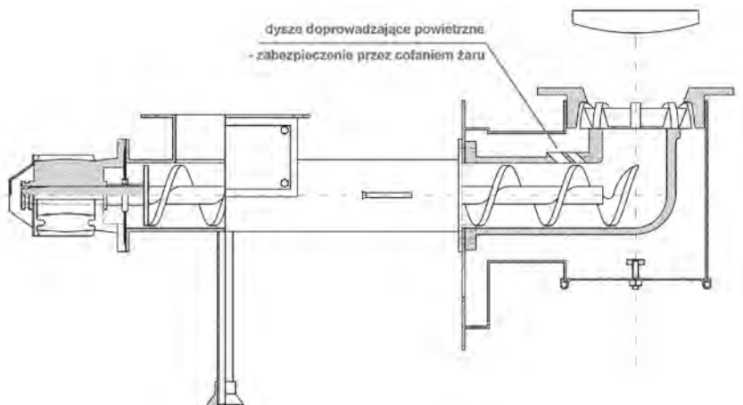
Rysunek 10 Retorta z dyszami powietrznymi zabezpieczającymi przed cofaniem żaru.
