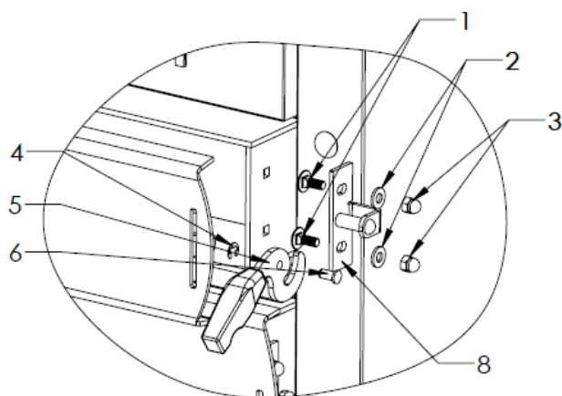
Rys.4a. Rączka drzwiczek i bolec blokujący
