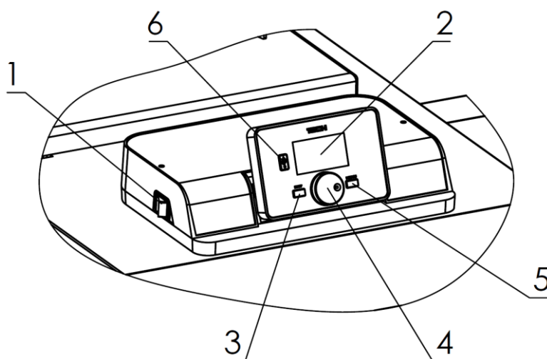
Rys. 2. Panel sterujący sterownika EL 483 zPID
