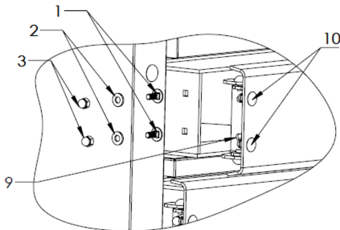
Rys.4b Zawias drzwiczek.
