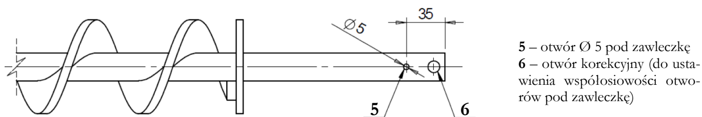
Rys. 21a. Demontaż ślimaka z podajnika kotła. palnika retortowego
