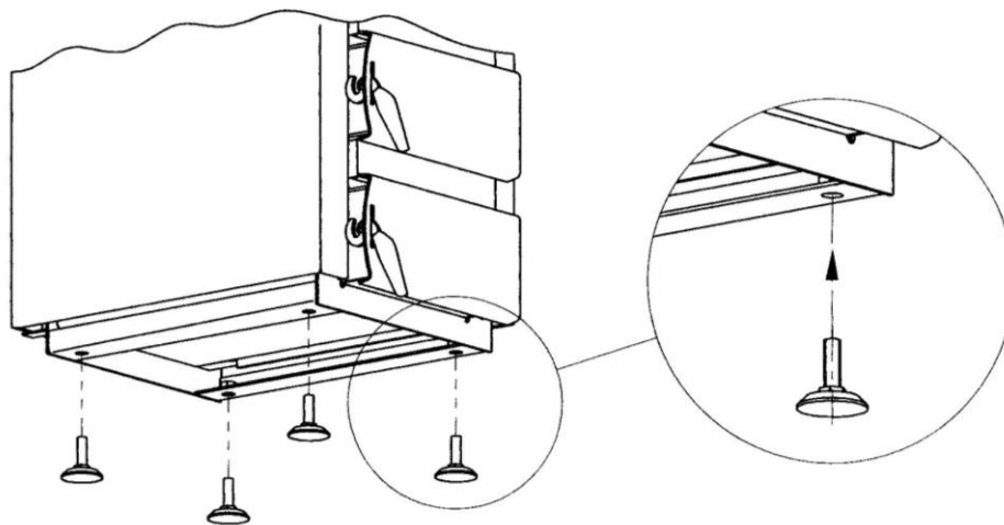
Rys. 5. Poziomowanie kotła
