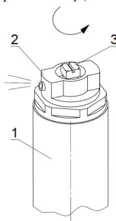
Rys.10. Odpowietrznik
