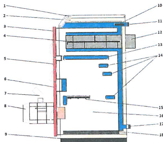
Przekrój wzdłużny kotła HEITZ BIO 34
