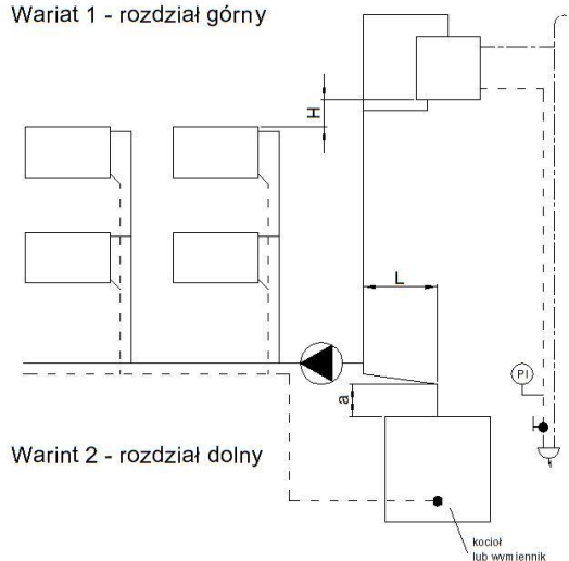
Rysunek 1a
