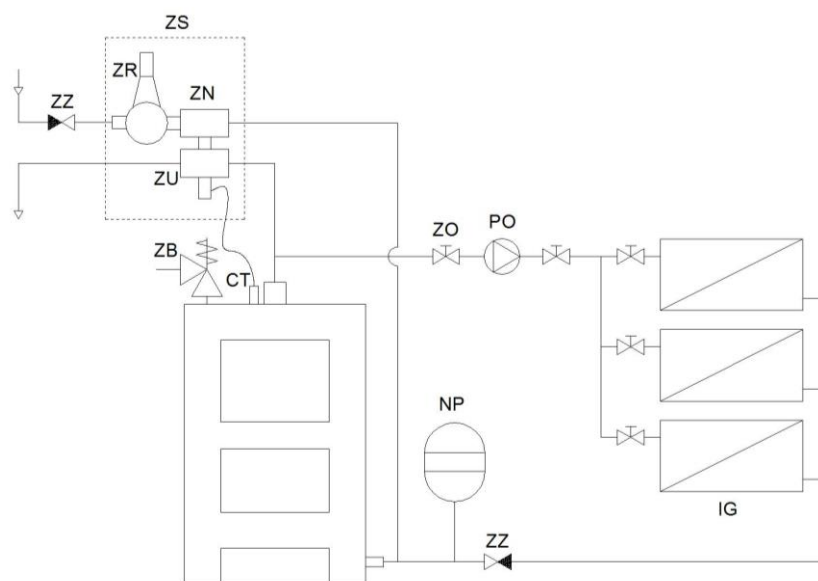
Rys. 3. Schemat montażu kotła w układzie zamkniętym zabezpieczony zaworem schładzającym.
