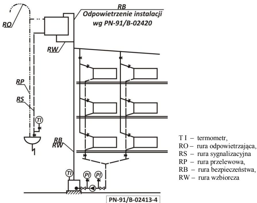
Rys.4 Schemat zabezpieczenia instalacji ogrzewania wodnego, wyposażonej w jeden kocioł lub wymiennik ciepła, rozdział górny, pompa zamontowana na powrocie.
