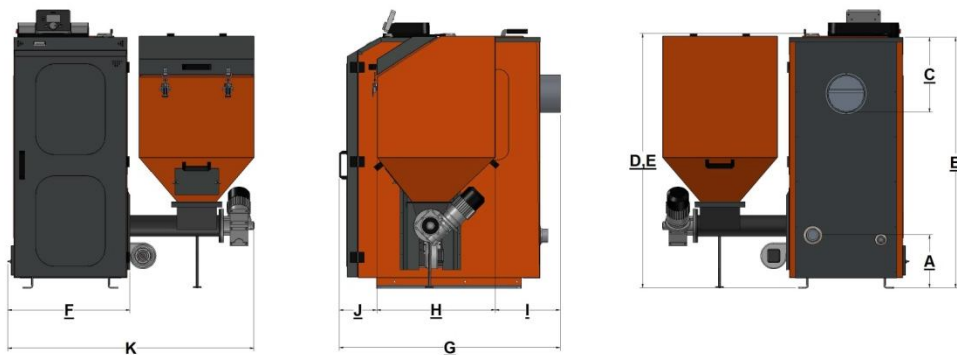
Rys. 2 Podstawowe wymiary kotłów AQUA ECO 17 kW i 25 kW z osprzętem ( patrz tab. nr 3 )
