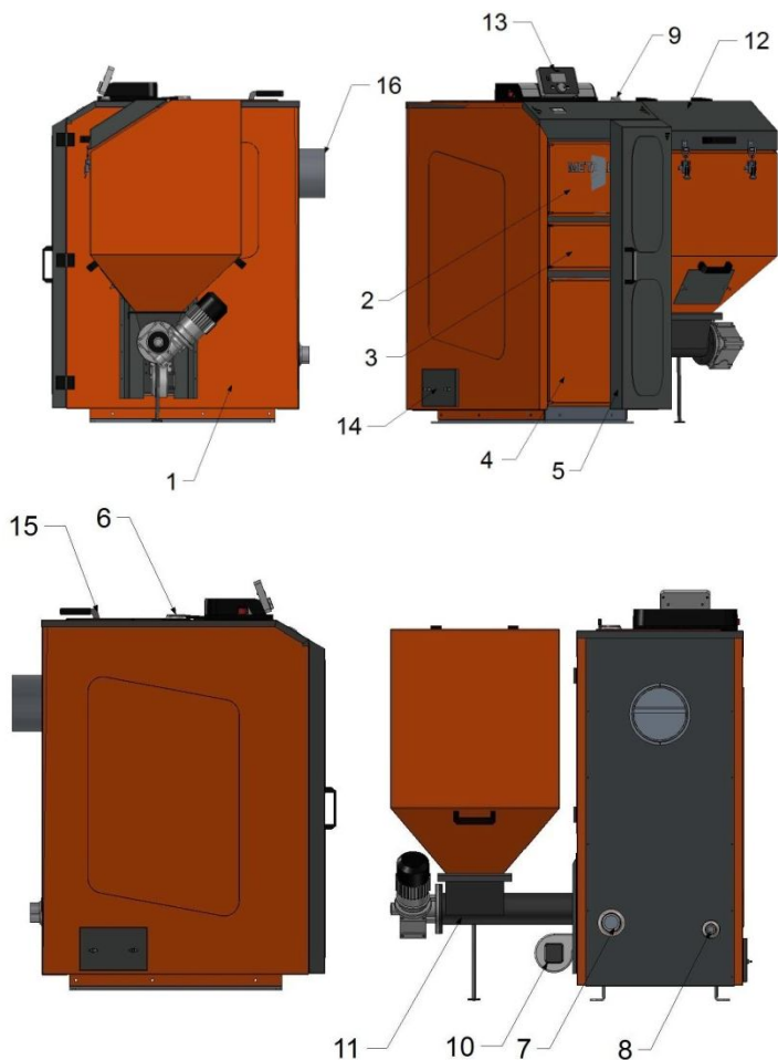
Rys.1 Podstawowe elementy kotłów AQUA ECO 17 kW i 25 kW z osprzętem;
