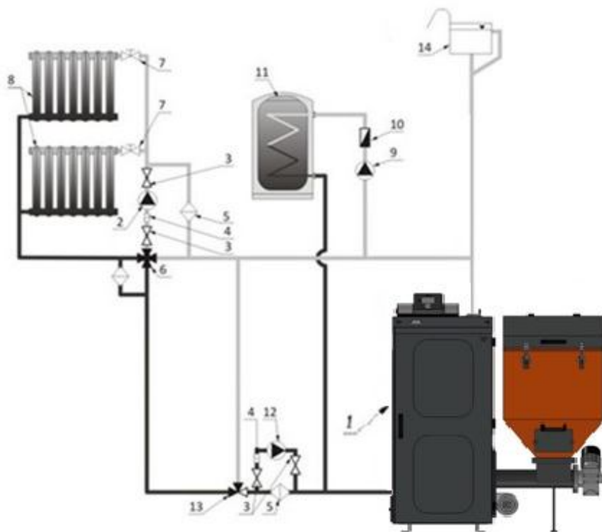
Rys. 10 Przykładowy schemat instalacji grzewczej systemu otwartego
