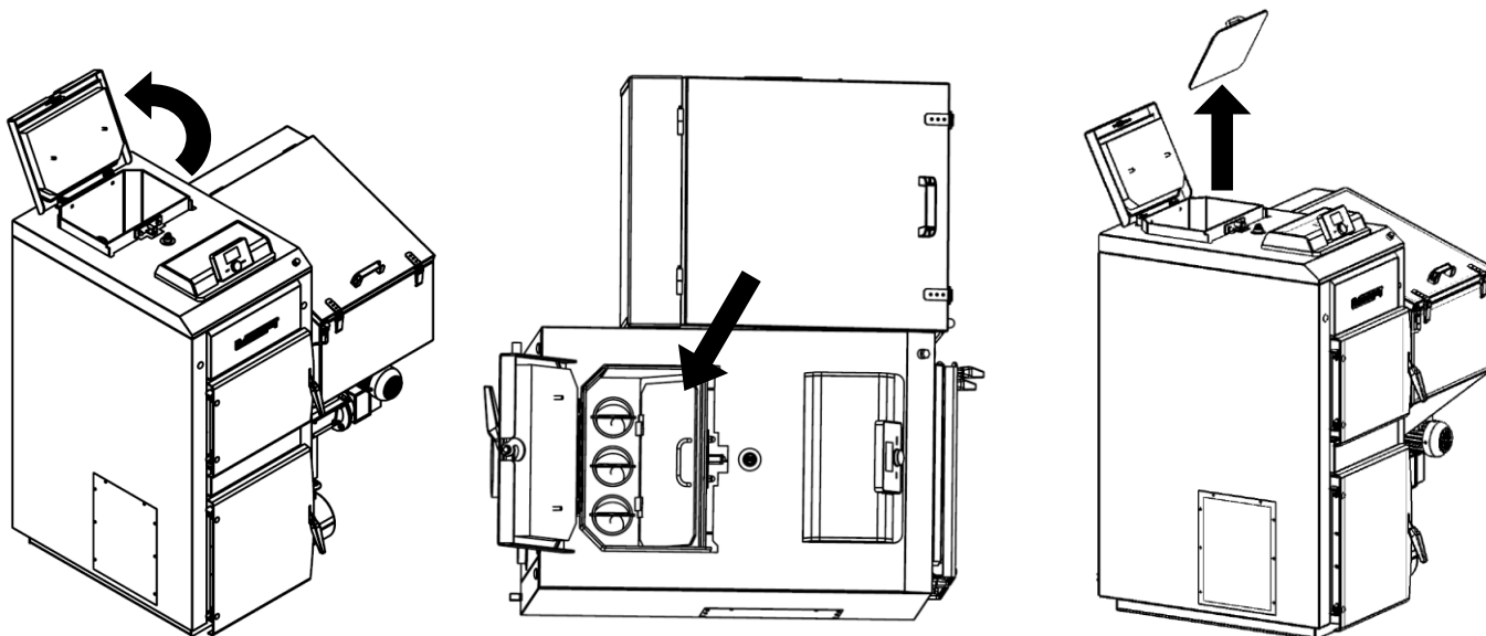
Rys. 14a. Otwarcie wyczystki górnej i wyciągnięcie klapy kierownicy ciągu.
