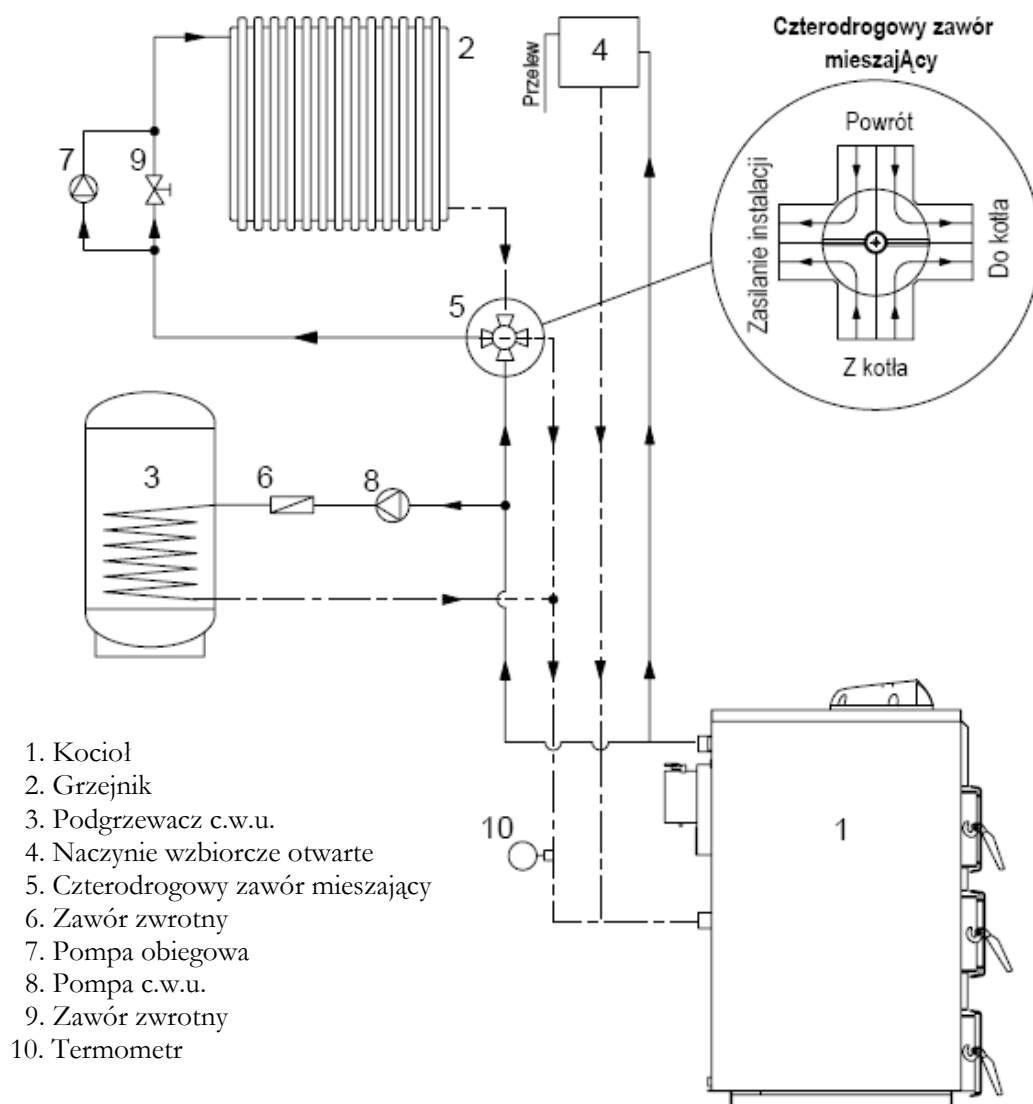
Rys. 12. Przykładowy schemat podłączenia kotła do systemu grzewczego c.o. i c.w.u. z wykorzystaniem czterodrożnego zaworu mieszającego.
