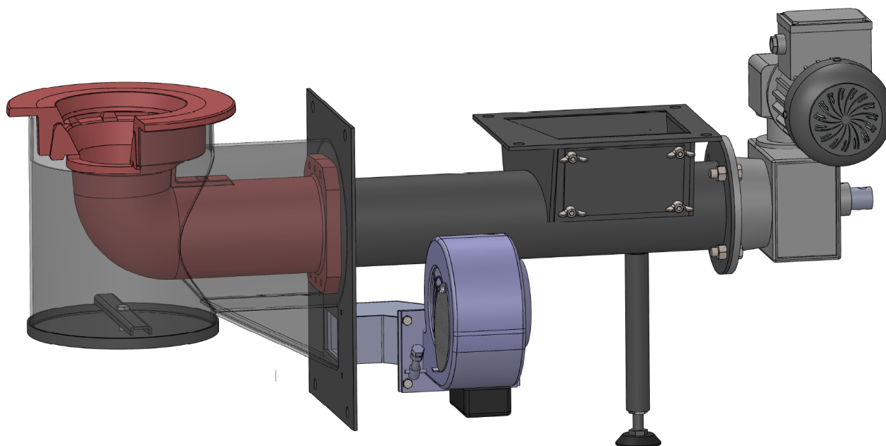
Rys. 17. Pogląd układu podawania i spalania paliwa
