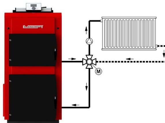
Rys.10a. Przykład montażu zaworu mieszającego czterodrogowego.
