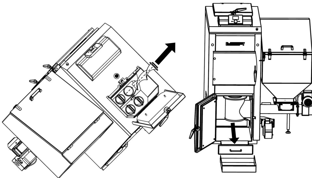
Rys. 14b. Widok na tylni wymiennik rurowy. Wyciągnięcie turbilatorów oraz popielnika rur konwekcyjnych.
