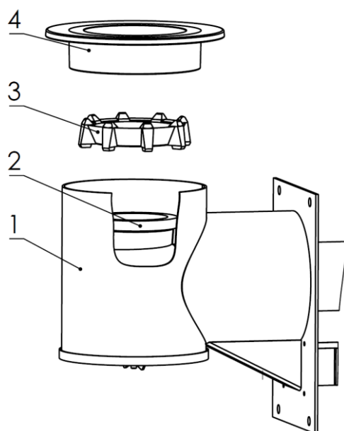
Rys. 15a. Demontaż palnika retortowego
