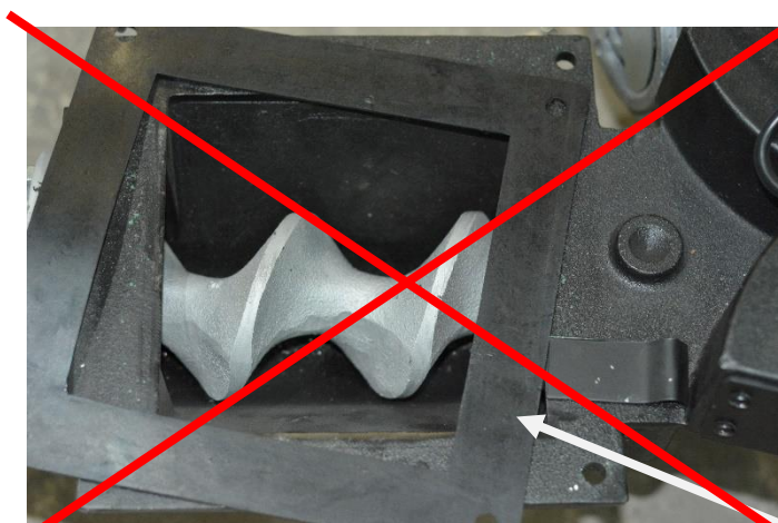
Rys. Na uchwyt nakładamy gumową uszczelkę (pamiętaj o dopasowaniu uszczelki do ramki podajnika) lub uszczelniaacz kominkowy
