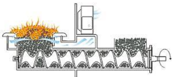
Rys. Prawidłowy poziom paliwa na palenisku retortowym
