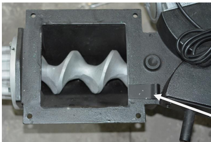
Rys. Na korpus podajnika nakładamy uchwyt czujnika
