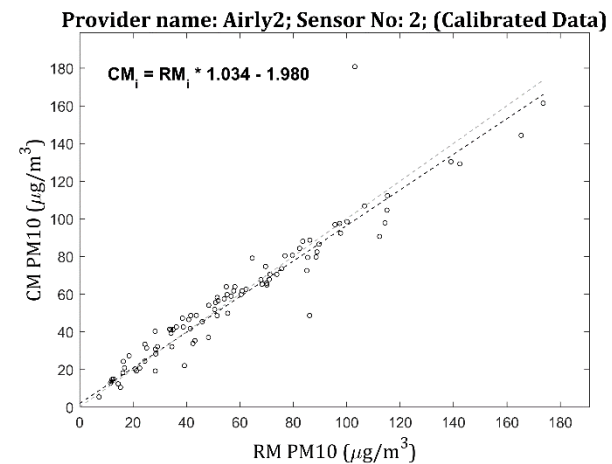
Rysunek 5.2. Krzywe korelacji pomiędzy wartościami mierzonymi przez testowane urządzenia (CM) dostarczone przez firmę Airly B a metodyką referencyjną (RM) dla frakcji PM 10 , niezależnie dla obu testowanych czujników (panel lewy czujnik nr 1, panel prawy czujnik nr 2). Na górnych wykresach przedstawiono zależności przed dokonaniem kalibracji urządzeń, na dolnych po wykonaniu kalibracji. Czarnymi okręgami przedstawiono wartości mierzone, czarną linią przerywaną - krzywą regresji liniowej ( CM = B \cdot RM + A ), szarą linią przerywaną - relację tożsamościową ( CM = RM ).
