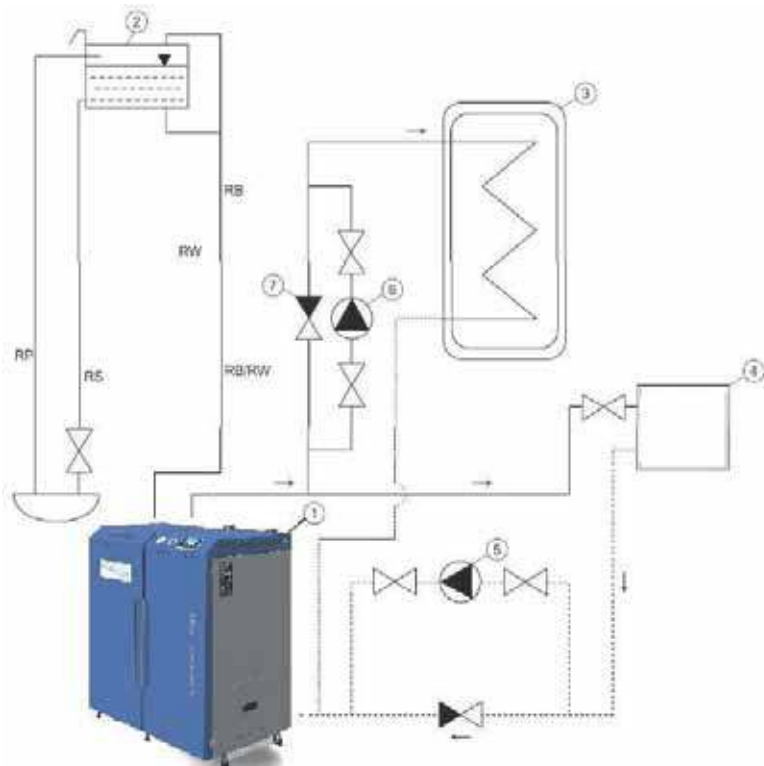
Rys. 4. Schemat poglądowy zabezpieczenia kotła DWOREK BIO COMFORT BLUE w układzie grzewczym otwartym, gdzie: 1 – kocioł, 2 – naczynie wzbiorcze (przelewowe), 3 – zasobnik c.w.u., 4 – obieg grzewczy, 5 – pompa c.o. (obiegowa), 6 – pompa c.w.u. (obiegowa), 7 – zawór różnicowy, RO – rura odpowietrzająca, RS – rura sygnalizacyjna, RB – rura bezpieczeństwa, RW – rura wzbiorcza, RP – rura przelewowa
