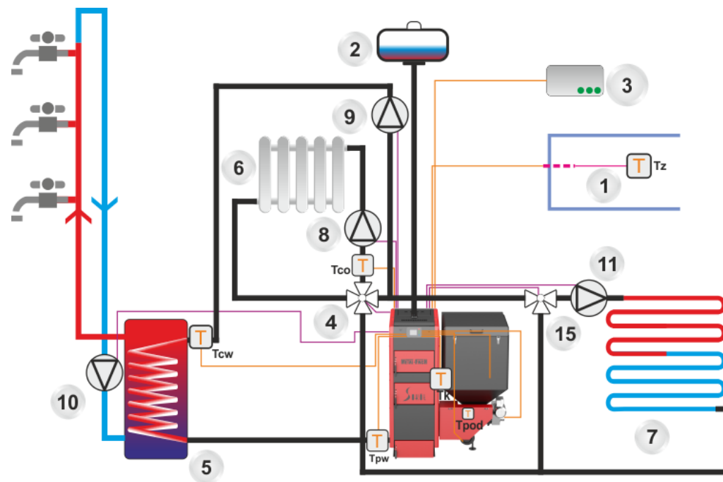
Rysunek 13.3 Podłączenie kotła do instalacji grzewczej
