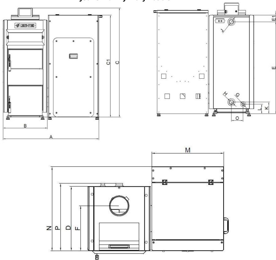
Rysunek 7.1 Wymiary kotła SMART PELLET
