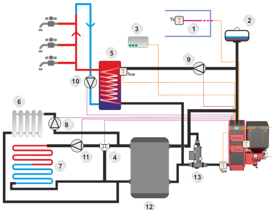
Rysunek 13.4 Podłączenie kotła do instalacji grzewczej z laddomatem i buforem
