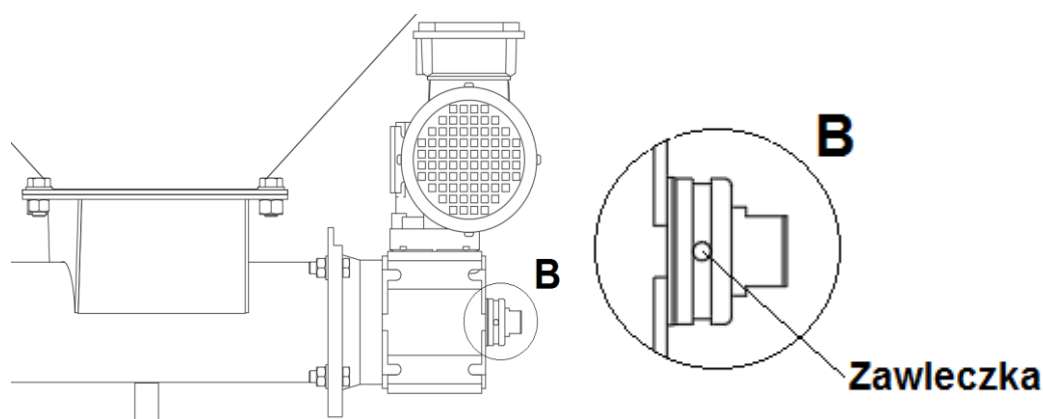
Rys. 7 Sposób montażu zawlecza motoreduktora ze ślimakiem
