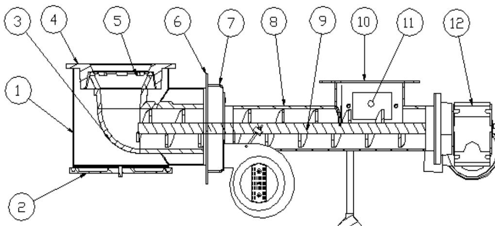
Rys.7 Budowa podajnika paliwa stałego
