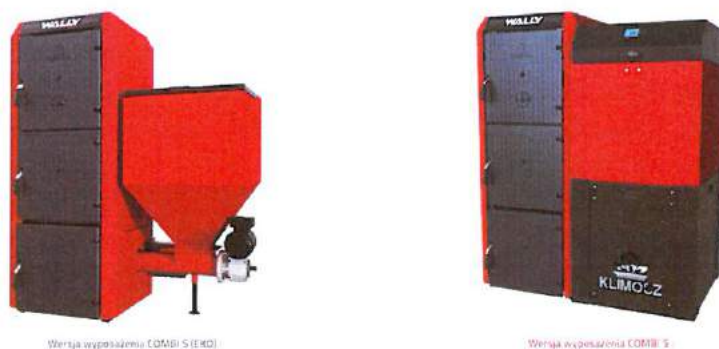
Rysunek 2. Rysunek poglądowy kotła Klimosz Combi S5 w wersji EKO (po lewej) i standard (po prawej).
