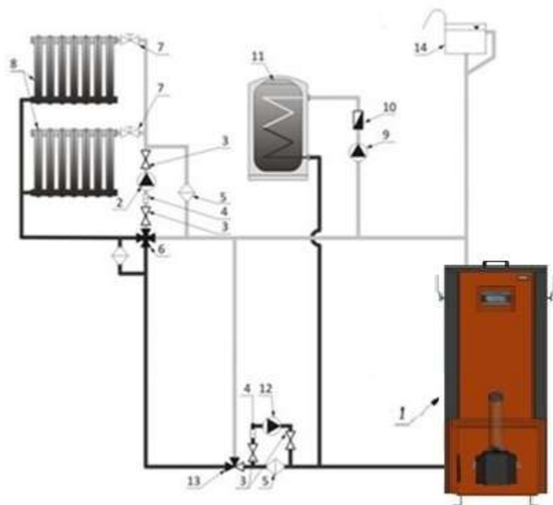
Rys. 10 Przykładowy schemat instalacji grzewczej systemu otwartego
