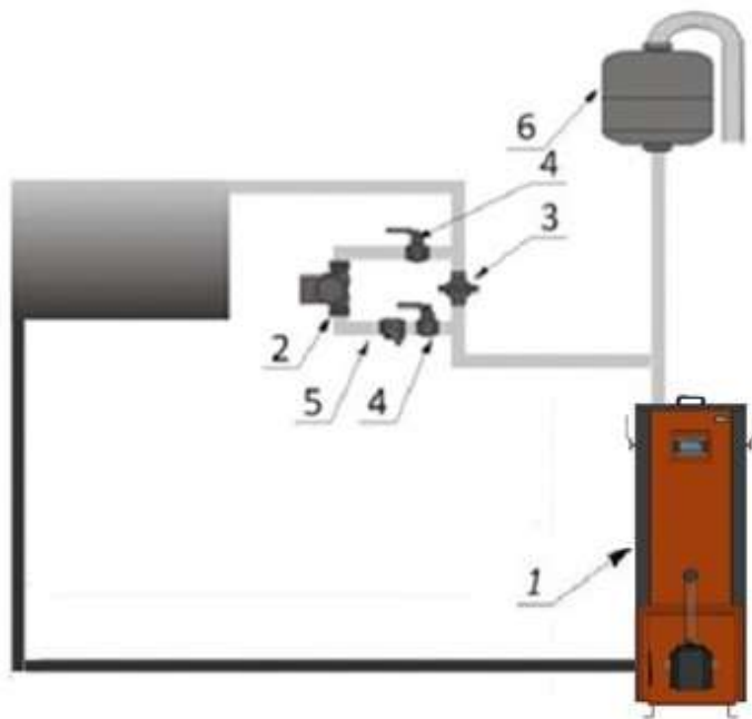
Rys. 5 Wykonanie obejścia grawitacyjnego:
