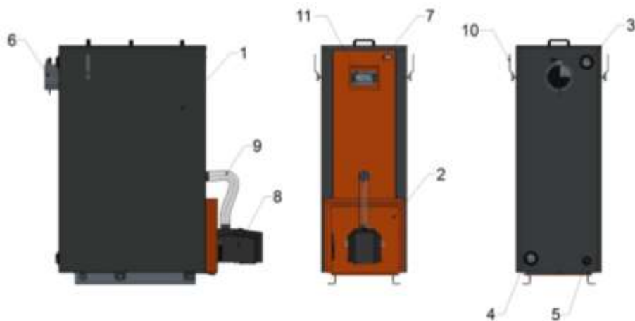
Rys.1 Podstawowe elementy kotłów typu ECO DELUX 11 kW ÷ 31 kW z osprzętem;
