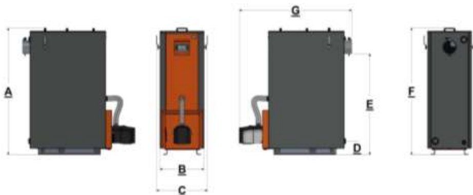
Rys. 2 Podstawowe wymiary kotłów typu ECO DELUX 11 kW ÷ 31 kW z osprzętem ( patrz tab. nr 3 )
