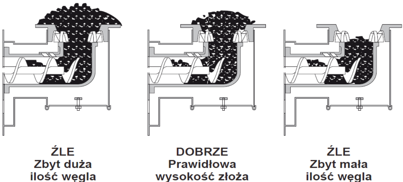
Rysunek 4. Prawidłowy poziom węgla na retorcie.
