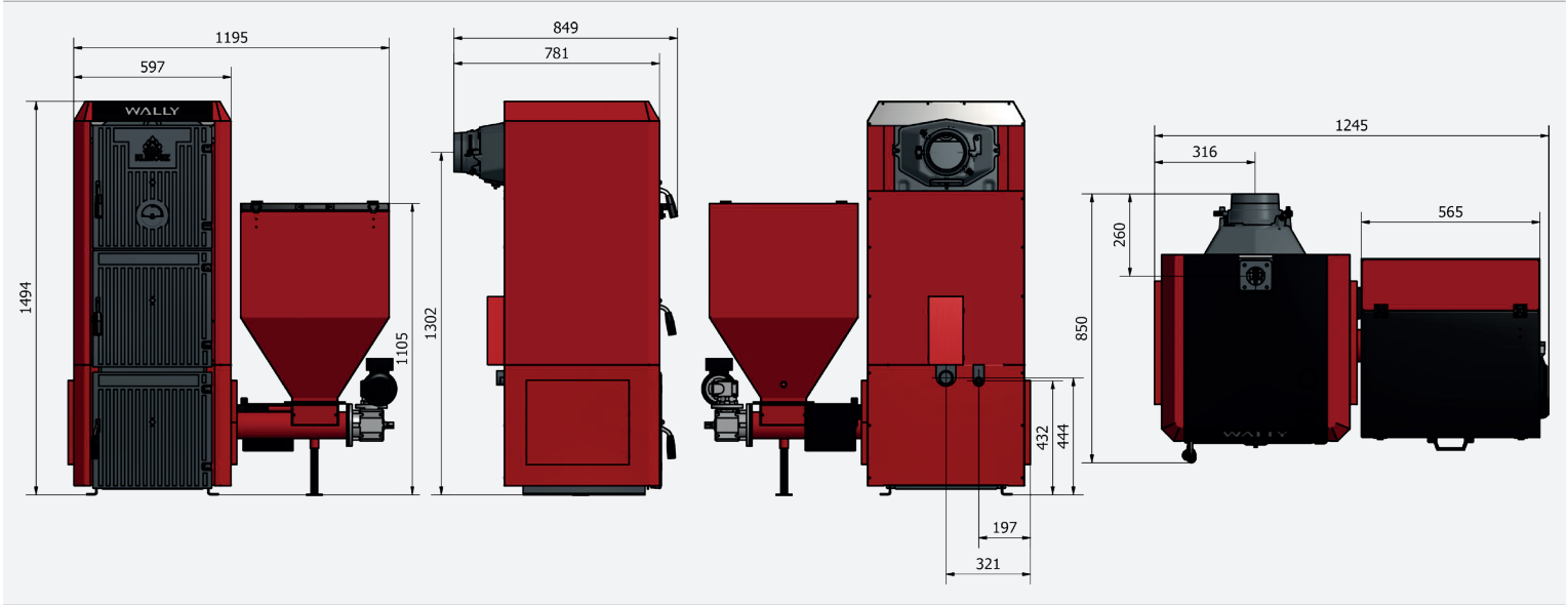
Wymiary KLIMOSZ COMBI S4 - wersja EKO
