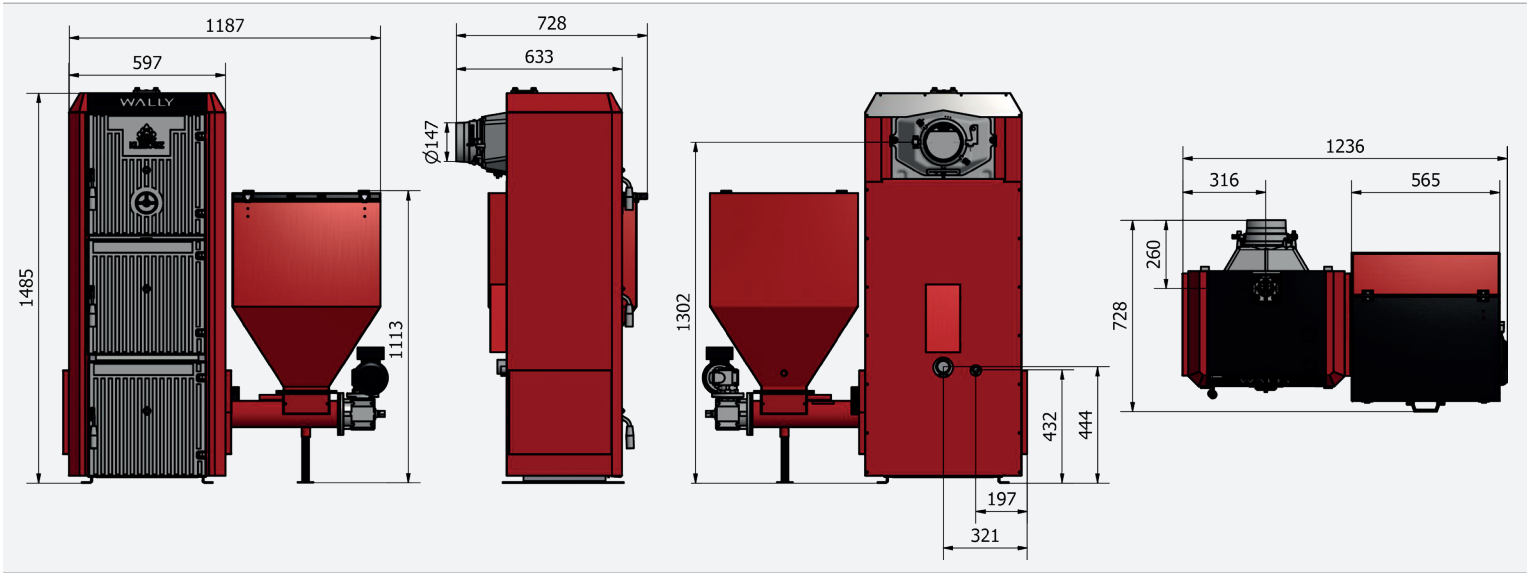
Wymiary KLIMOSZ COMBI S3 - wersja EKO
