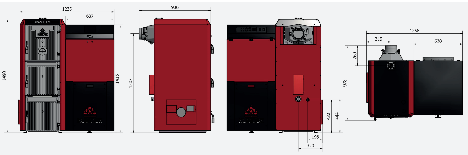
Wymiary KLIMOSZ COMBI S5 - wersja NG
