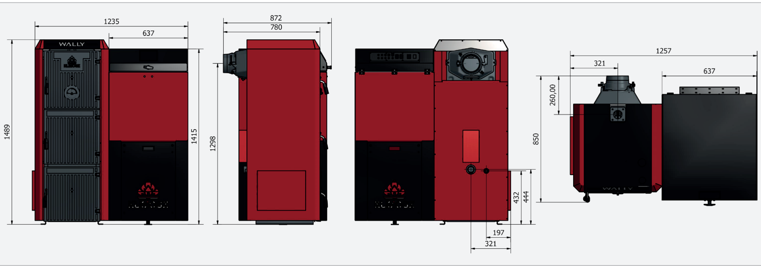
Wymiary KLIMOSZ COMBI S4 - wersja NG
