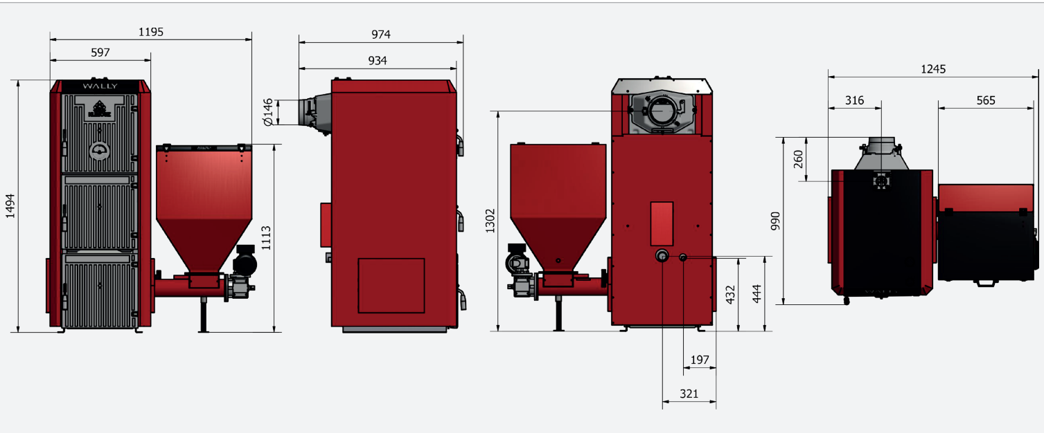
Wymiary KLIMOSZ COMBI S5 - wersja EKO
