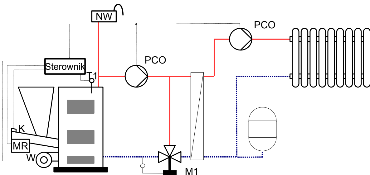
Rysunek przedstawia schemat podłączenia kotła w układzie otwartym z instalacją grzewczą pracującą w układzie zamkniętym. Obie instalacje połączone są wymiennikiem ciepła. Funkcję ochrony powrotu pełni zawór stałonastawny mieszający.
