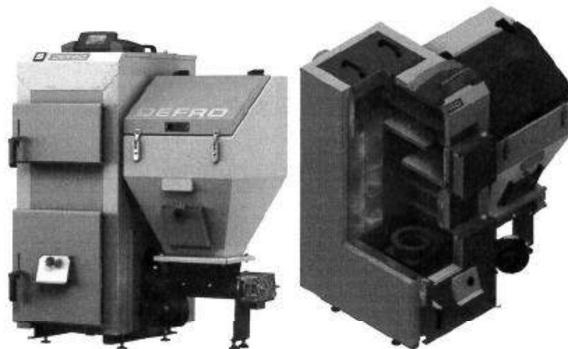
Rys. 1. Kocioł grzewczy wodny typu Sigma.
