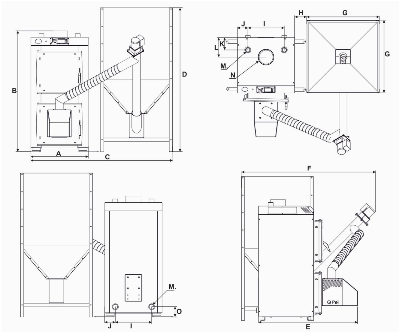
Rys.3.2.2.Wymiary kotłów sztoker®bio 12 – 24 kW.
