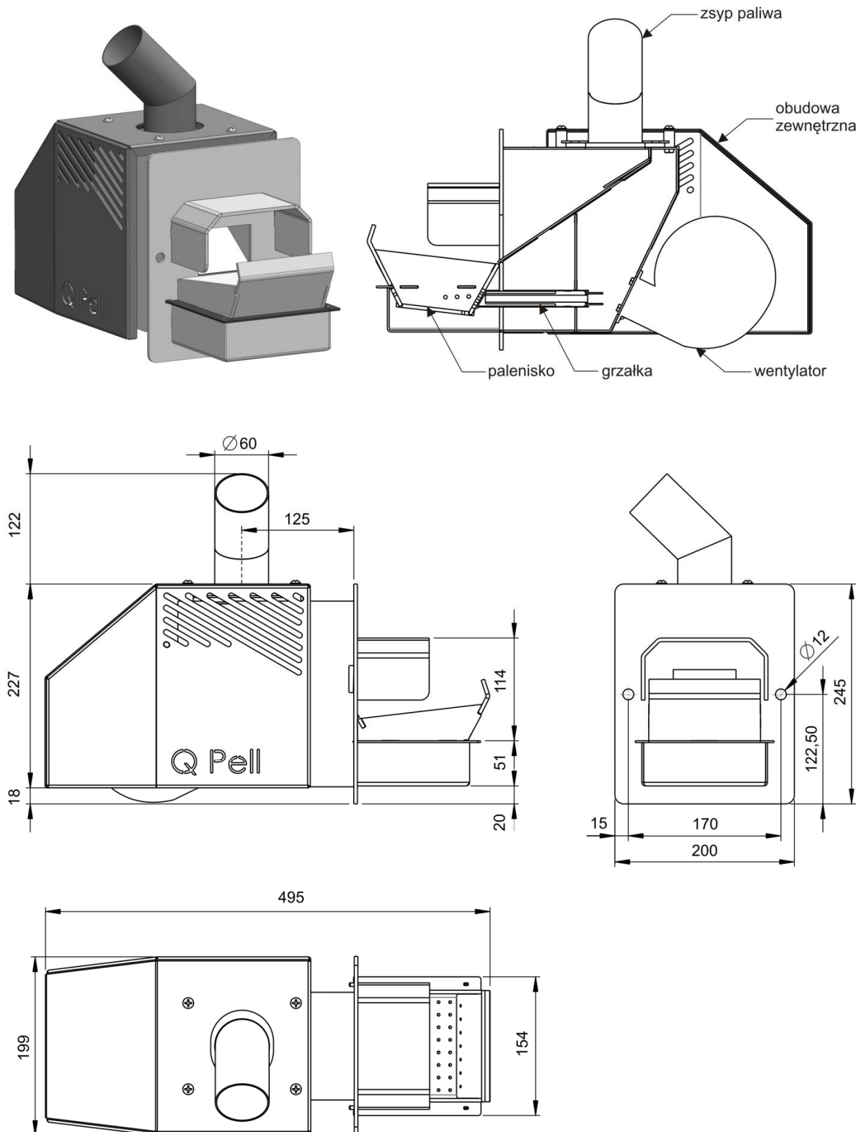
Rys.3.1.1.Przekrój ogólny i wymiary palnika QPel.
