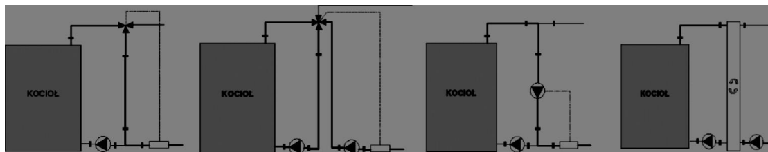
Rys. 2 Zalecane schematy połączeń kotła do instalacji grzewczej
