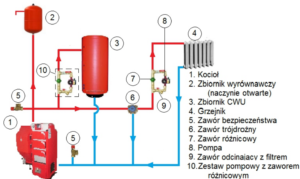
Rys. 2 Przykładowy schemat podłączenia kotła
