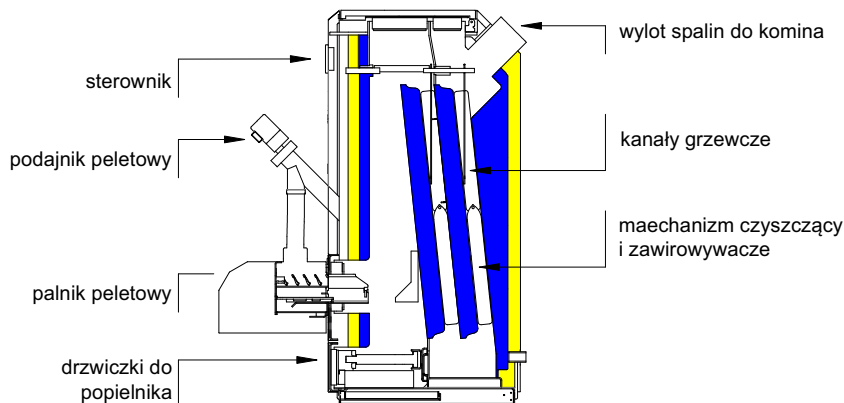
Rys. 1 Przekrój kotła
