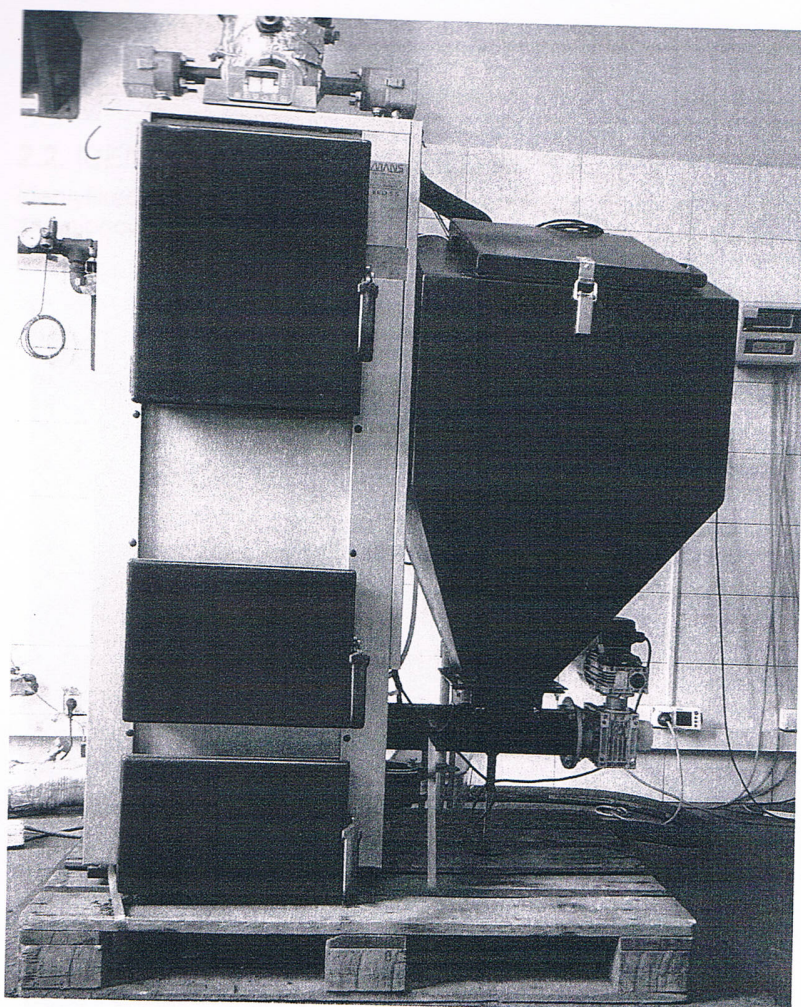
Rysunek 1. Fotografia kotła EKO 5 S
