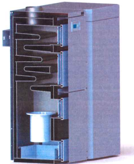
Rysunek 1. Wodny kocioł grzewczy typu DuoKo 24 kW.
