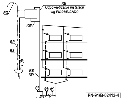
Rysunek 5. Schemat zabezpieczenia instalacji ogrzewania wodnego, wyposażonej w jeden kocioł lub wymiennik ciepła, rozdział górny, pompa zamontowana na powrocie. Schemat zabezpieczenia ma również zastosowanie do następujących instalacji ogrzewania wodnego:
