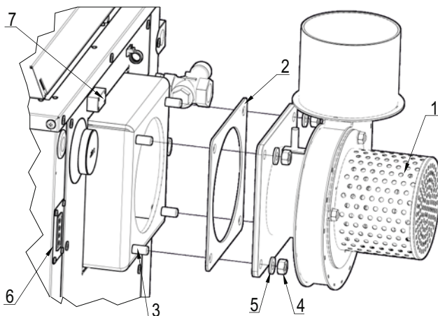
Rysunek 18. Instrukcja montażu wentylatora wyciągowego.
