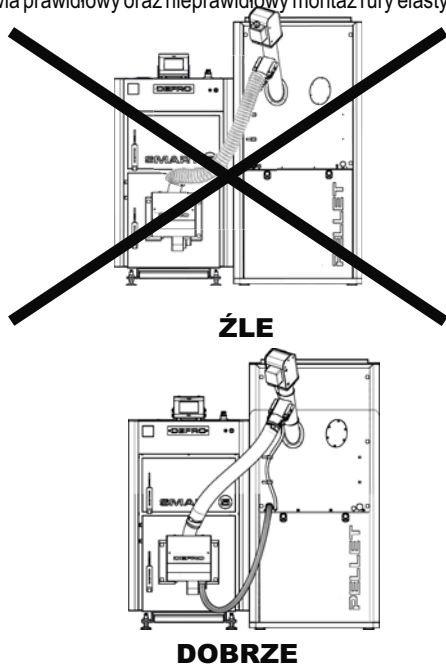
Rysunek 13. Prawidłowe ustawienie zasobnika paliwa względem kotła.
