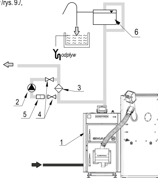
Rysunek 9. Wykonanie obejścia grawitacyjnego: 1-kocioł; 2-pompa obiegowa; 3-zawór różnicowy; 4-zawory odcinające; 5-filtr; 6-otwarte naczynie wzbiórcze.
