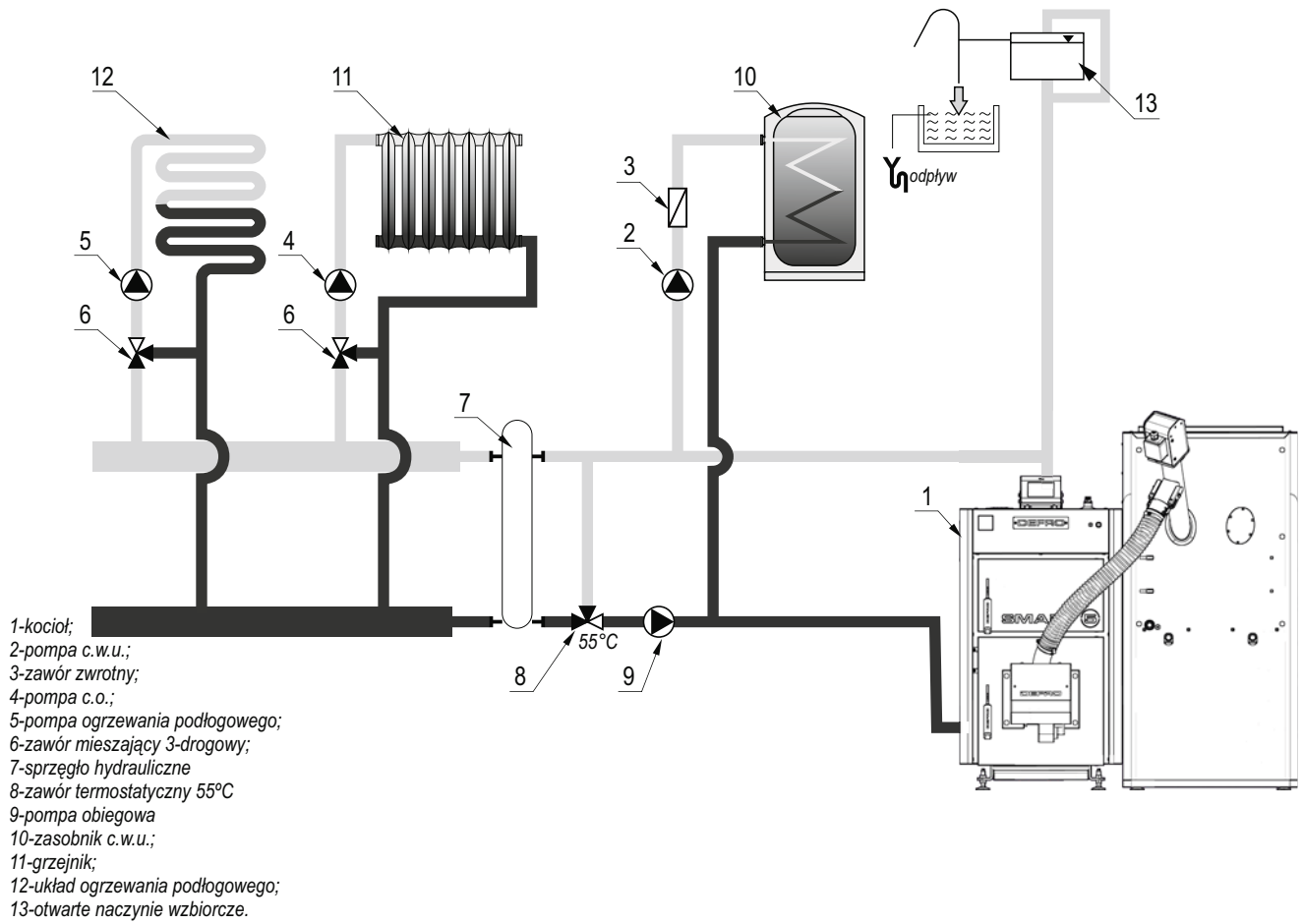
Rysunek 10. Uproszczony schemat instalacji grzewczej systemu otwartego.
