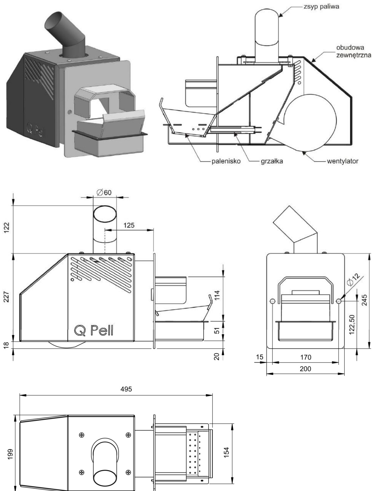
Rys.3.1.1.Przekrój ogólny i wymiary palnika QPell.
