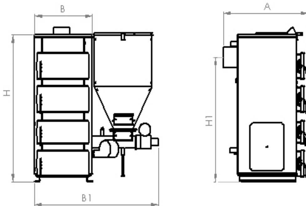
RYS. 2 Wymiary kotła V4
