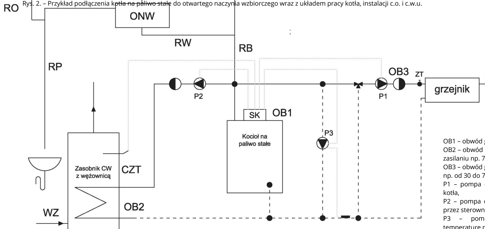
Rys. 2. – Przykład podłączenia kotła na paliwo stałe do otwartego naczynia wzbiorniczego wraz z układem pracy kotła, instalacji c.o. i c.w.u.
