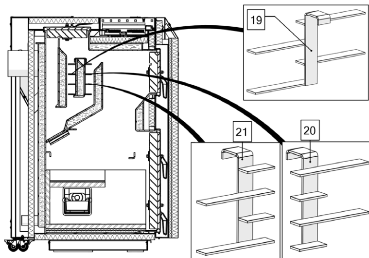
Rys.: Zestaw zaworowawczy oraz ich umiejscowienie w kotle Twin Bio Luxury Compact typ NE 8-12
