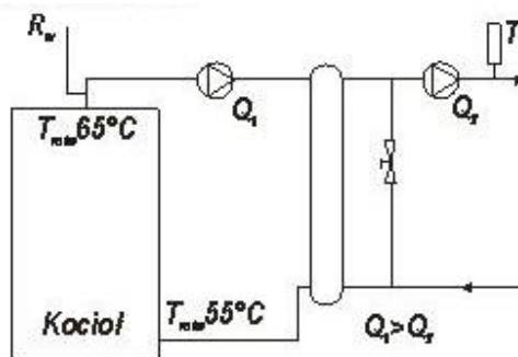
Rys. 8 Schemat połączenia kotła z instalacją grzewczą z wykorzystaniem sprzęgła wodnego.
